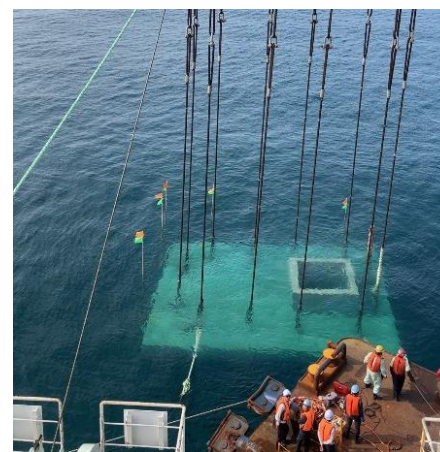
放水蓋設置作業の状況②
