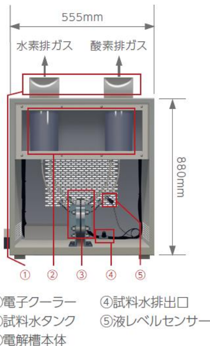
電解濃縮ユニット
