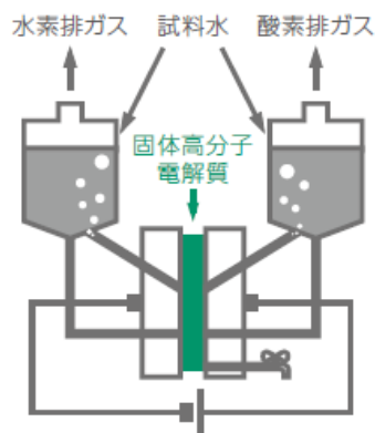
装置概略図
