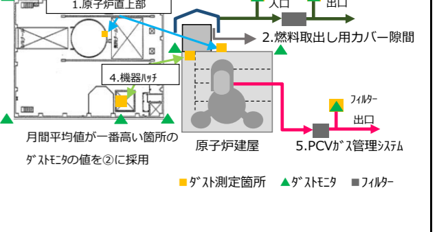
3号機原子炉建屋の開口部のイメージ 月間平均値が一番高い箇所のダストモニタの値を②に採用
