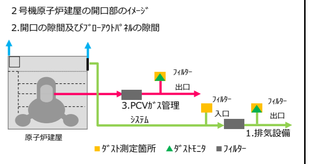
2号機原子炉建屋の開口部のイメージ 2. 開口の隙間及びBOP隙間
