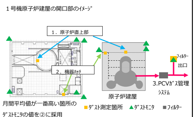
1号機原子炉建屋の開口部のイメージ 月間平均値が一番高い箇所のダストモニタの値を②に採用
