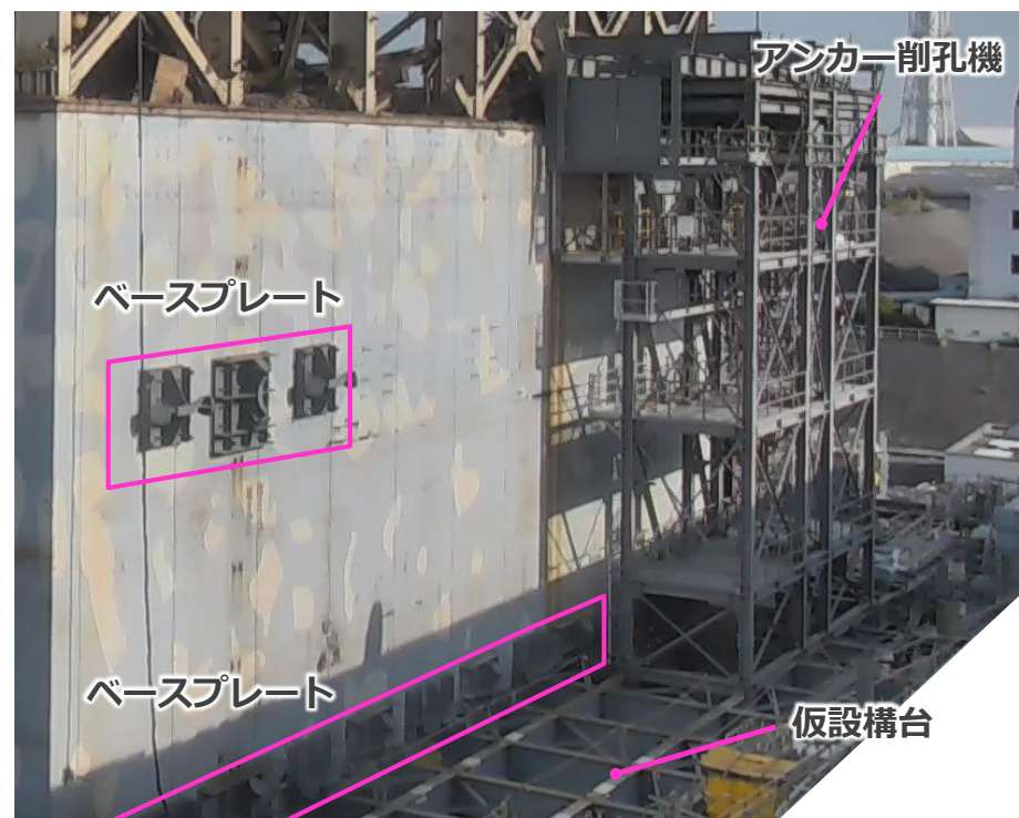
アンカー削孔状況 (東面) (撮影：2023年7月24日)
