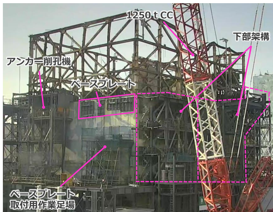
現場状況 (北西面) (撮影：2023年7月24日)
