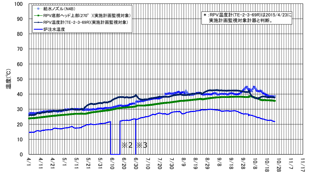
2号機 原子炉圧力容器まわり温度(4/1～10/24)
