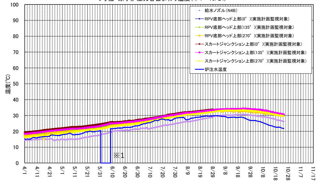
3号機 原子炉压力容器まわり温度(4/1~10/24)
