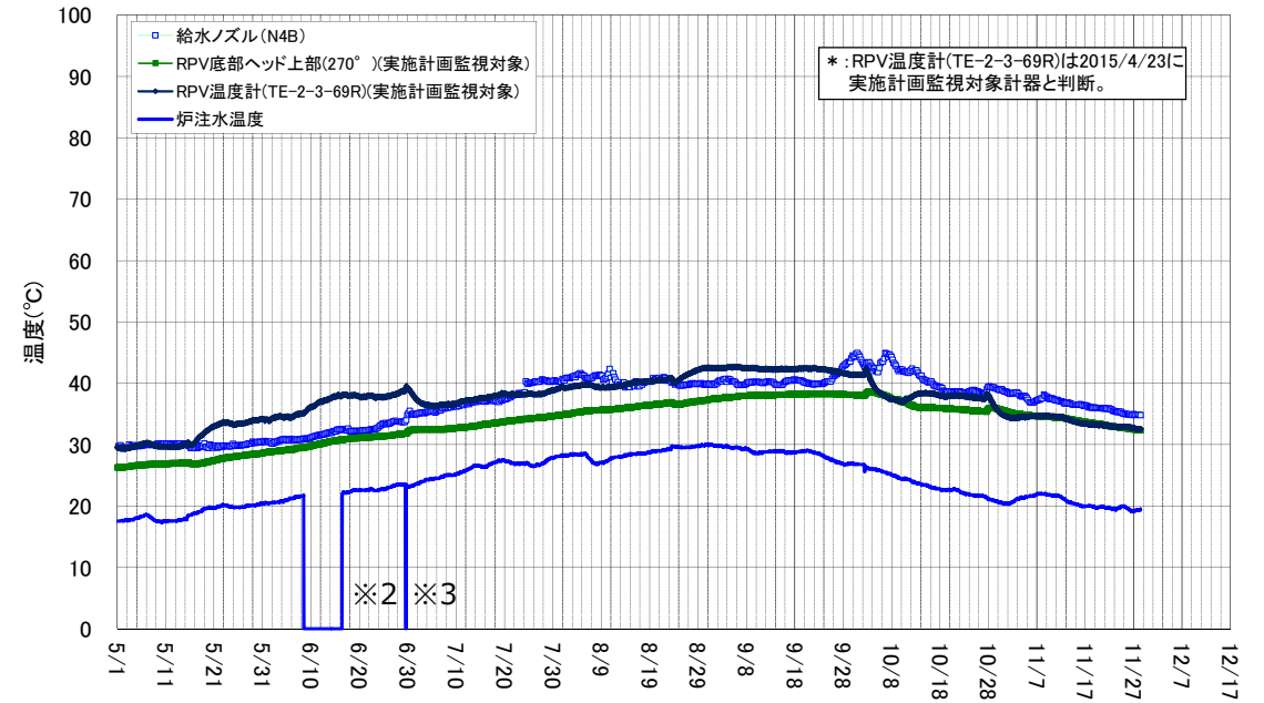
2号機 原子炉圧力容器まわり温度(5/1~11/28)
