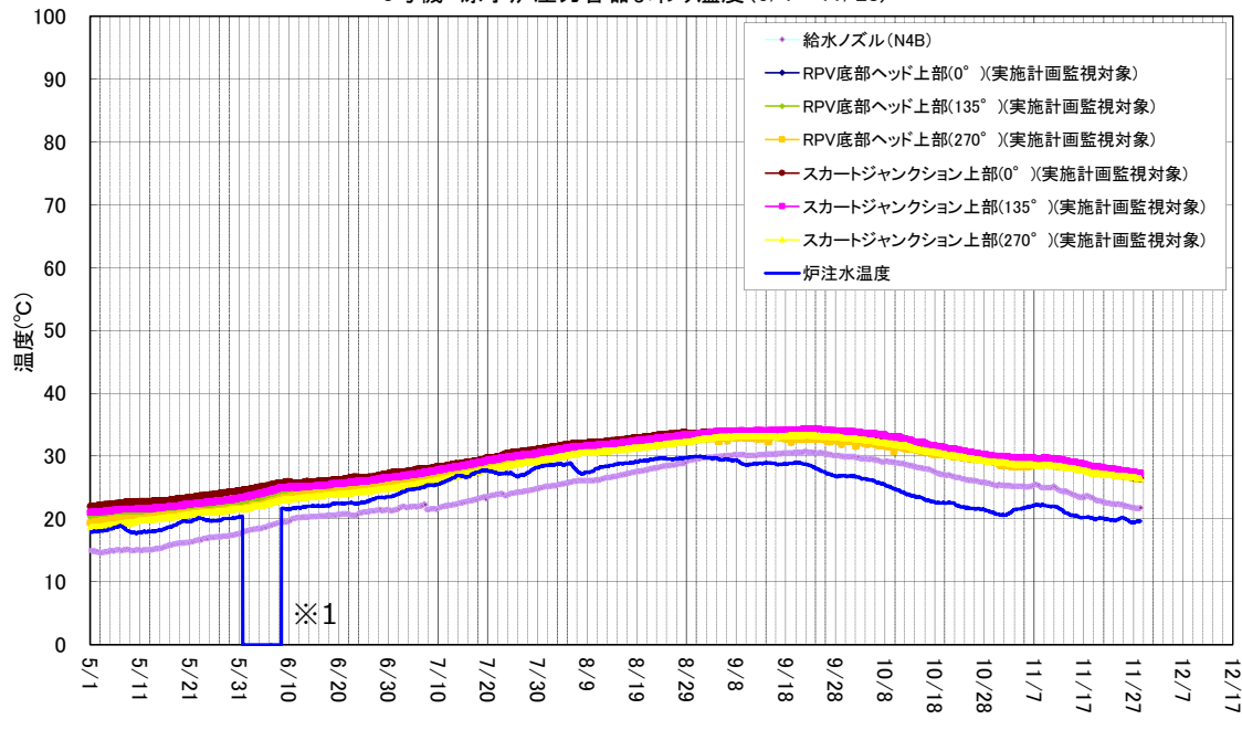
3号機 原子炉压力容器まわり温度 (5/1~11/28)
