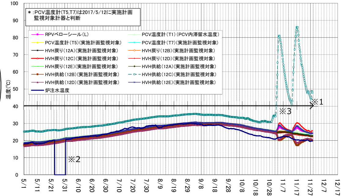
1号機 D/W雰囲気温度(5/1~11/28)
