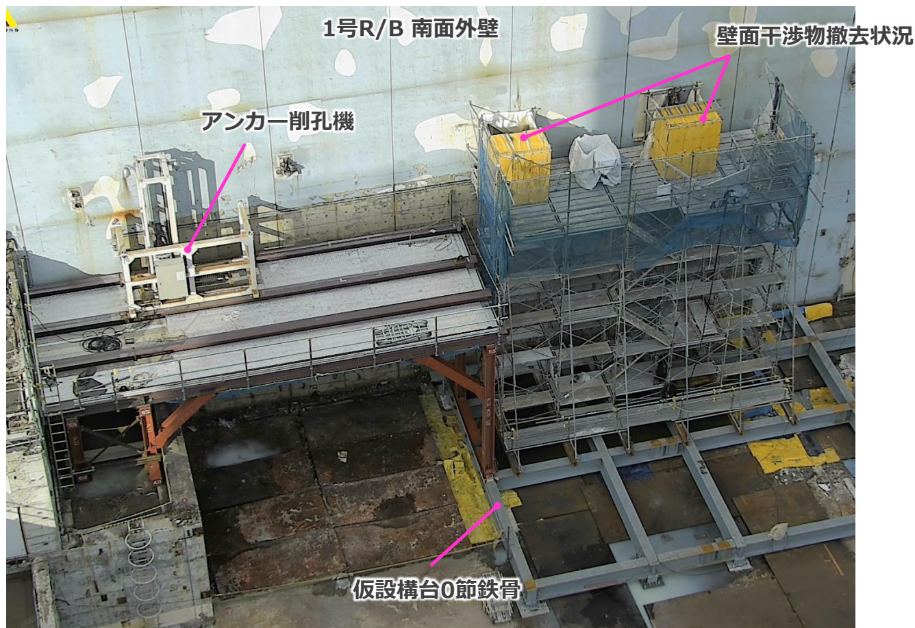
アンカー削孔・壁面干渉物撤去状況（1号機R/B 南側）
