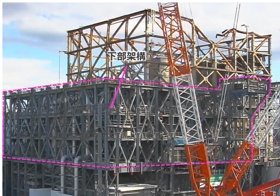
現場状況（北西面） （撮影：2023年11月28日）
