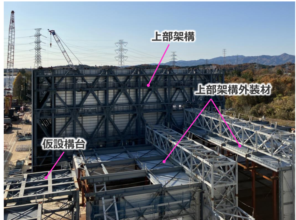
構外ヤード全景（撮影：2023年11月27日）
