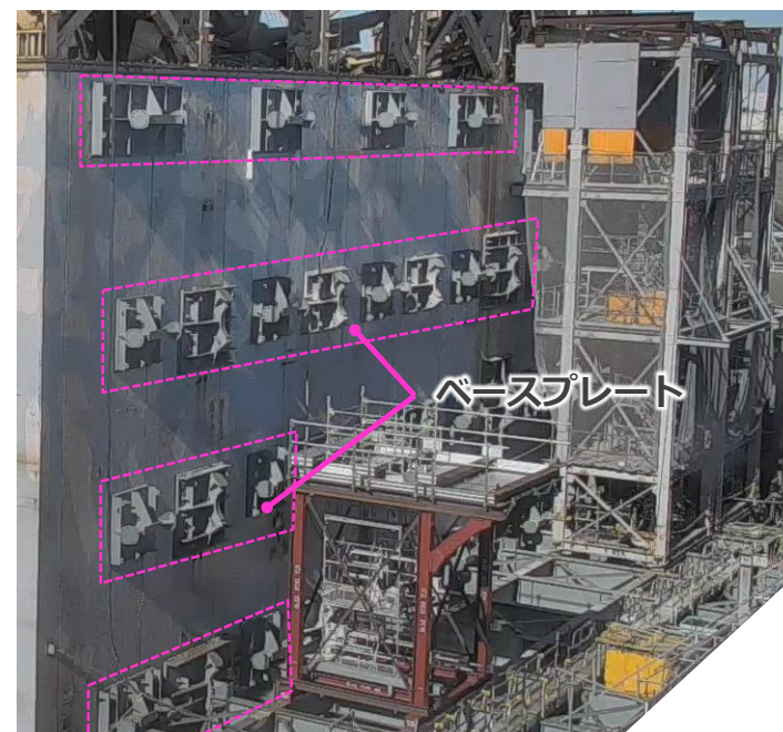
ベースプレート設置状況（東面） （撮影：2023年11月18日）
