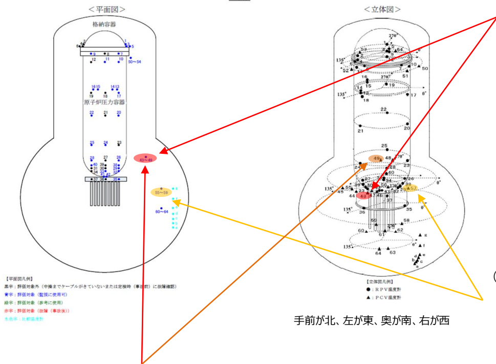
RPV/PCV温度計配置図
