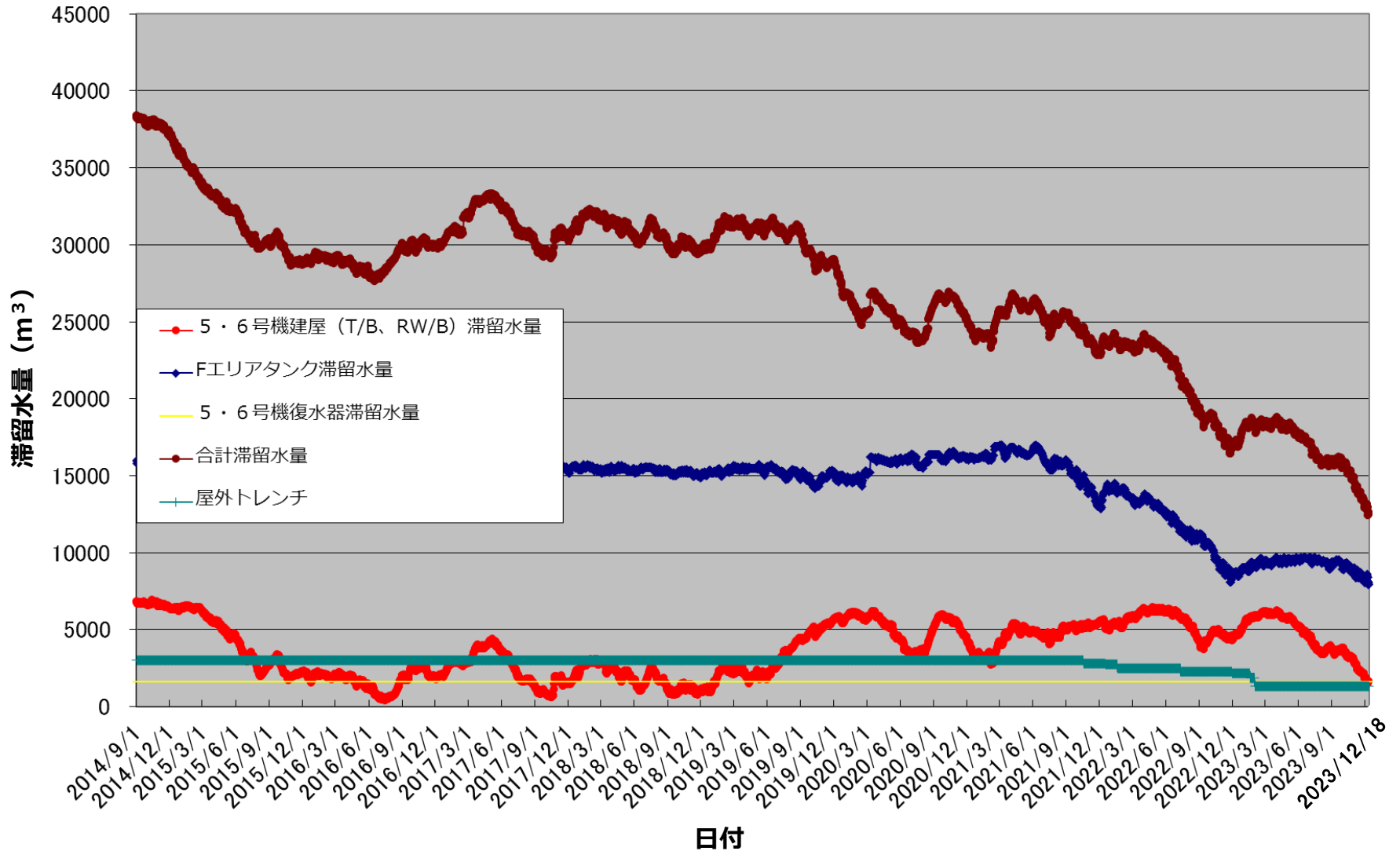
5・6号機 低レベル滞留水量の推移
