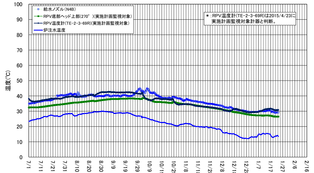
2号機 原子炉圧力容器まわり温度(7/1~1/23)
