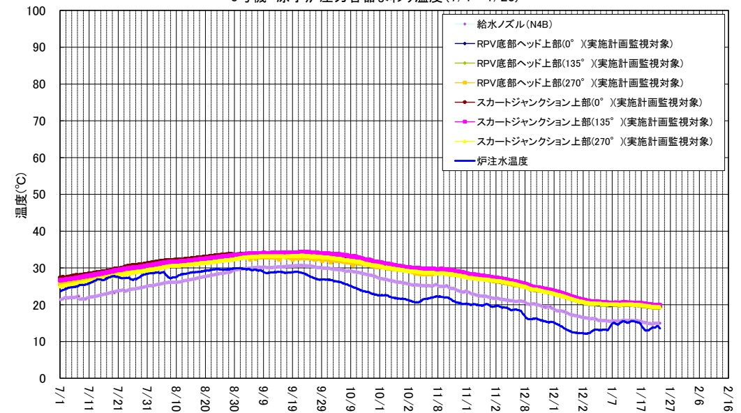
3号機 原子炉压力容器まわり温度(7/1~1/23)
