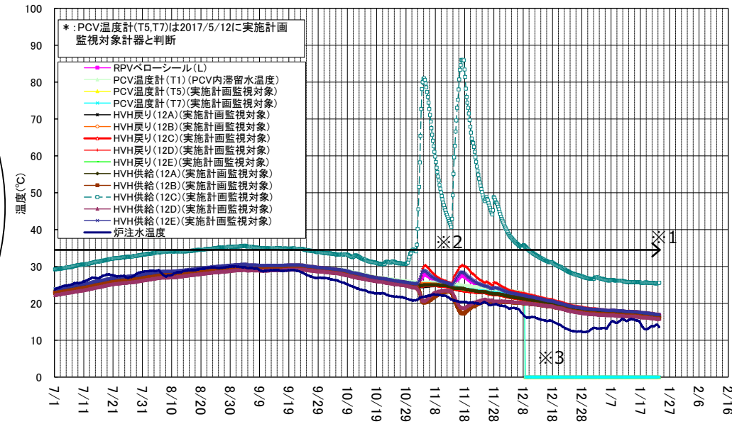
1号機 D/W雰囲気温度(7/1~1/23)
