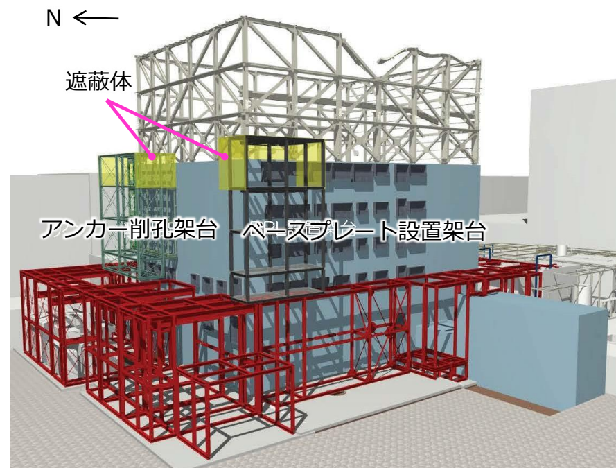
アンカー削孔架台・ベースプレート設置架台 への遮蔽体設置イメージ（北西面）
