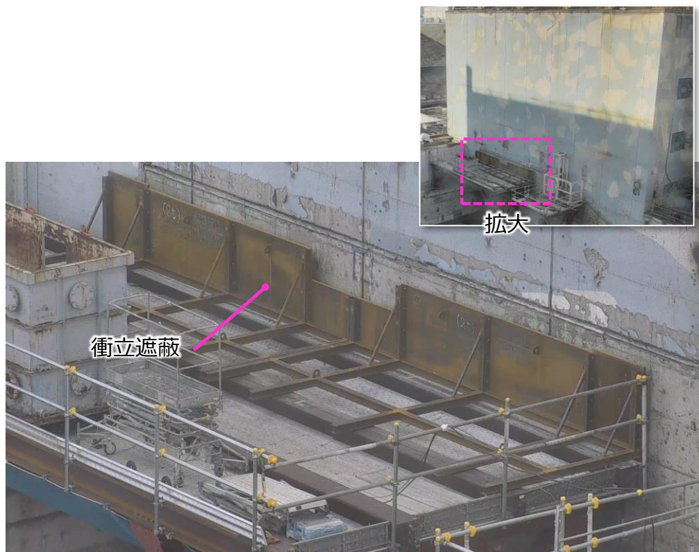
衝立遮蔽の設置状況（南面） (撮影：2024年1月24日)
