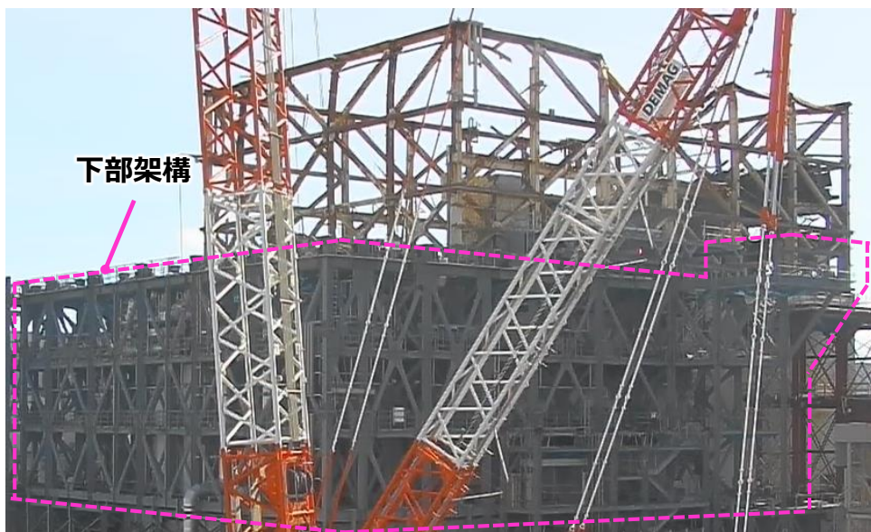
現場状況（北西面） (撮影：2024年1月24日)
