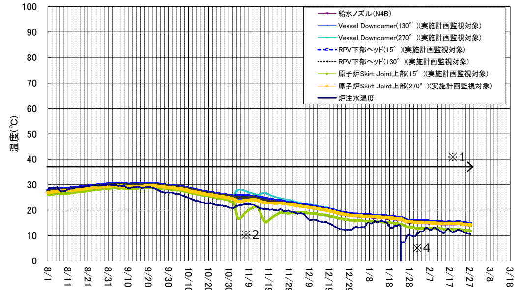
1号機 原子炉圧力容器まわり温度(8/1~2/27)
