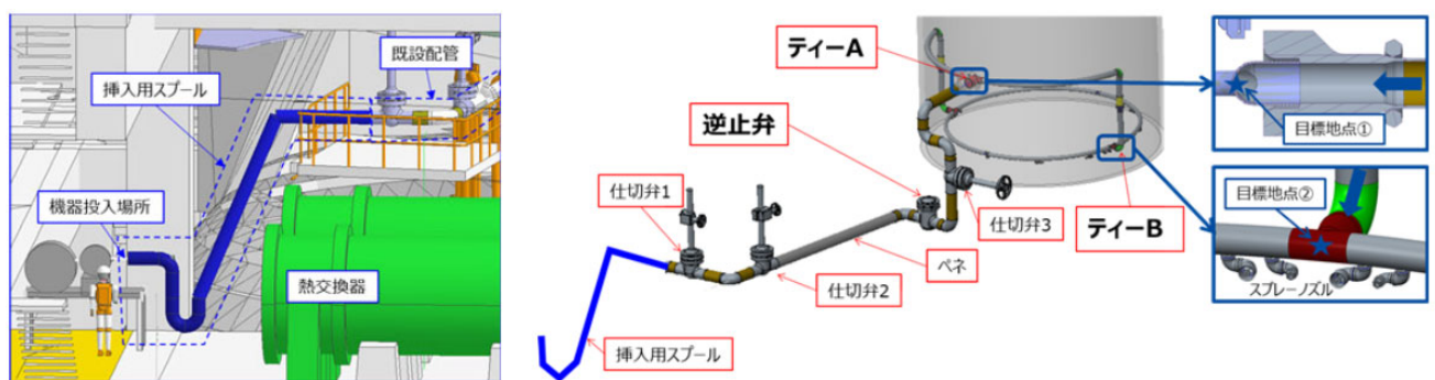
（炉心スプレー系配管アクセスルート）
