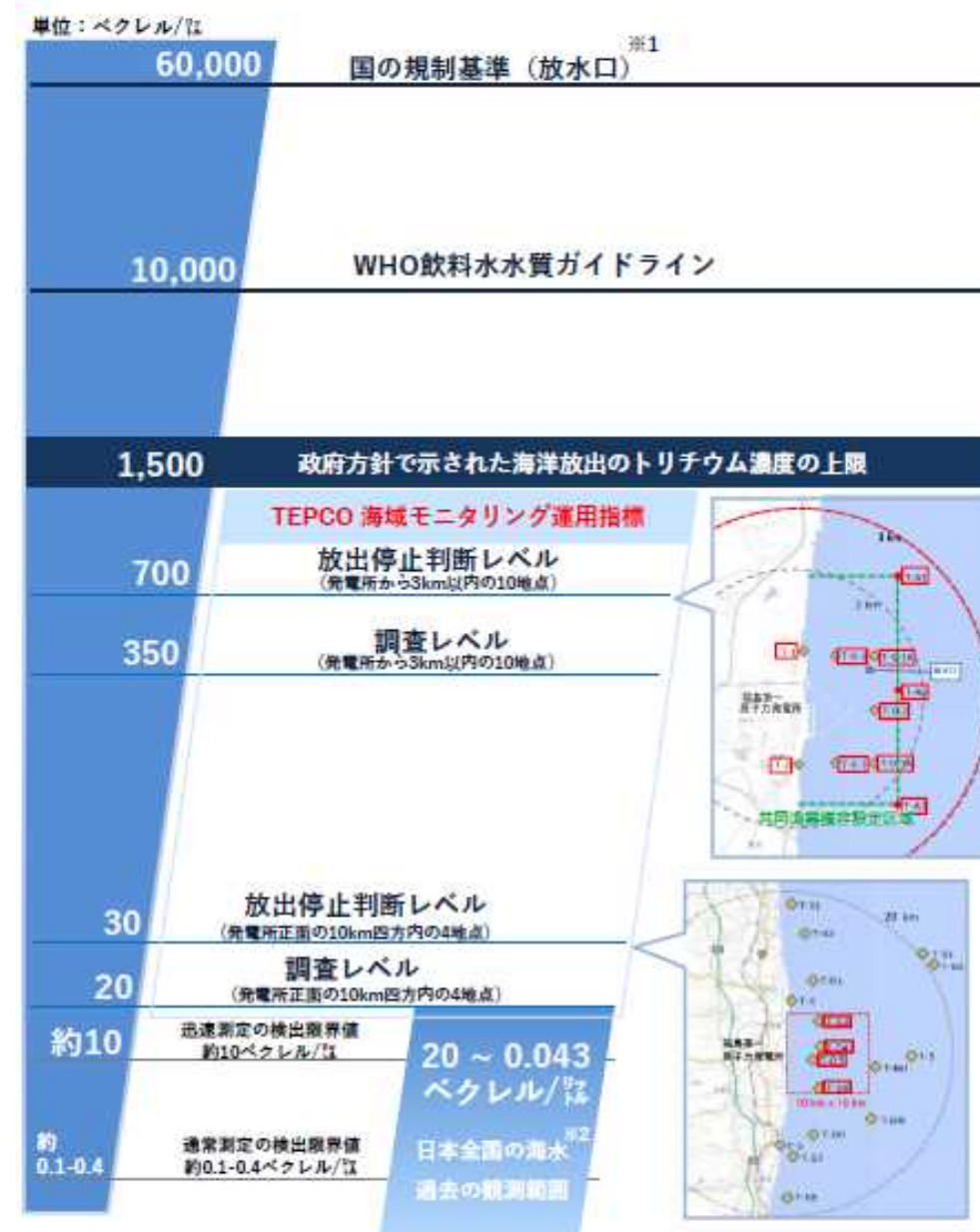
【参考】海水のトリチウム濃度の比較
