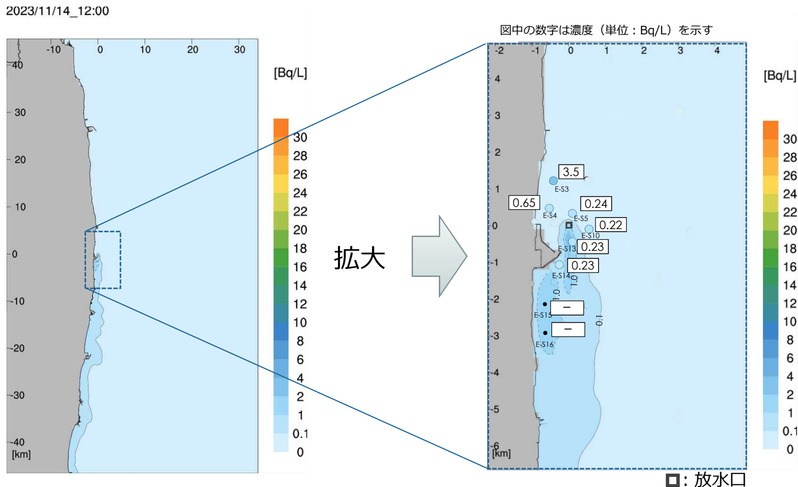
図 11月14日12:00の拡散計算結果（海表面の濃度分布図）とモニタリング結果の比較 ○の色はモニタリング結果の濃度を示し,白丸はND, ●はこの時間帯においてモニタリングを行っていないことを示す。
