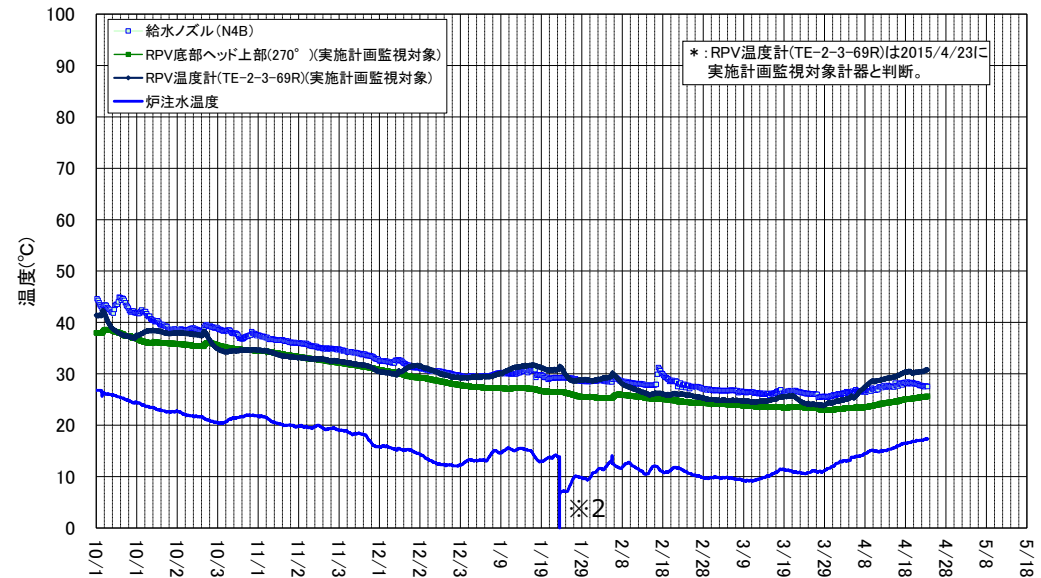
2号機 原子炉圧力容器まわり温度 (10/1～4/23)
