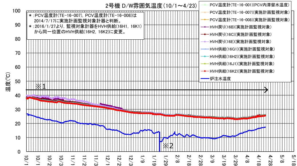
2号機 D/W雰囲気温度 (10/1～4/23)
