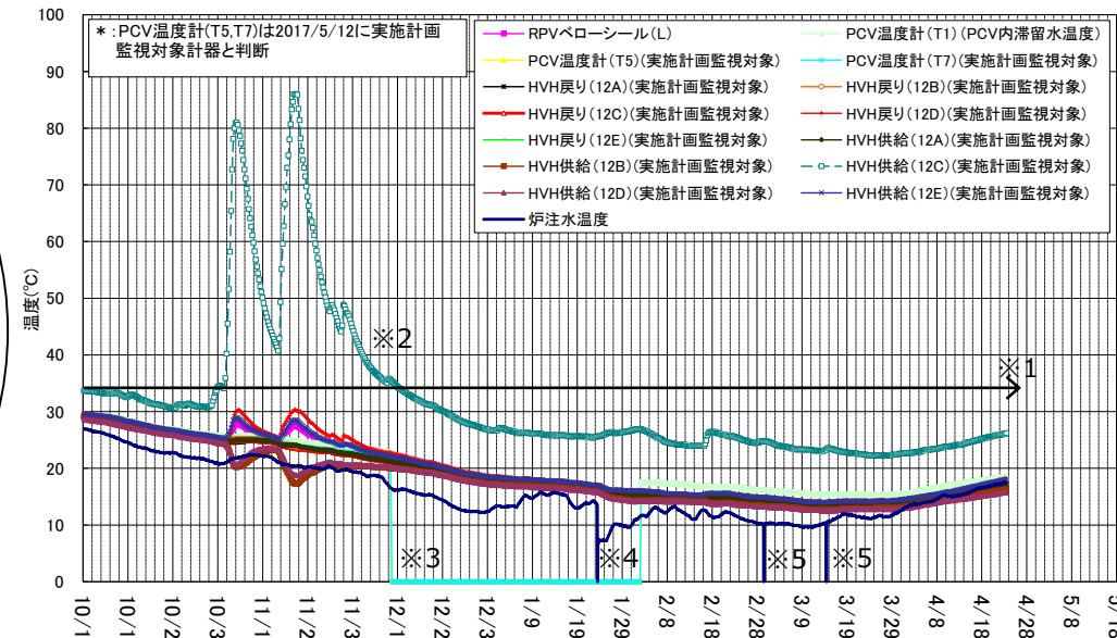
1号機 D/W雰囲気温度 (10/1～4/23)
