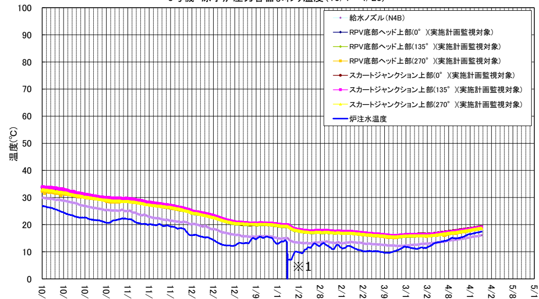
3号機 原子炉压力容器まわり温度 (10/1~4/23)
