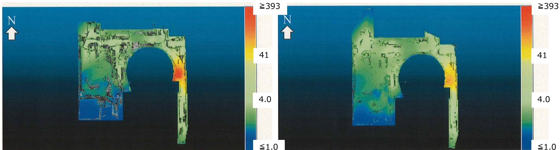
1号機R/B 3階 床上近傍0.20mの線量率分布 [mSv/h]
