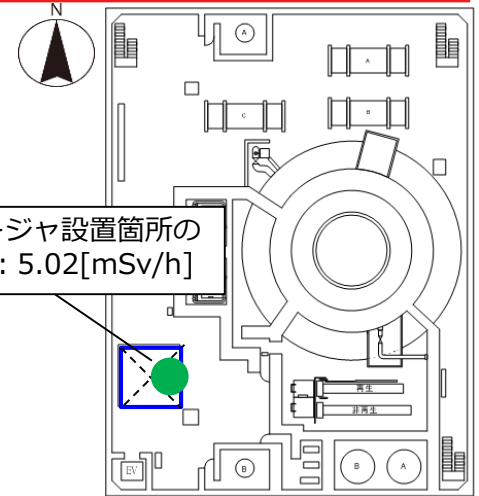
3号機R/B 2階
