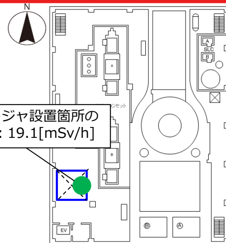
3号機R/B 4階
