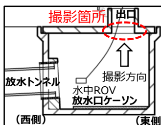
放水口ケーソン出口の状況
