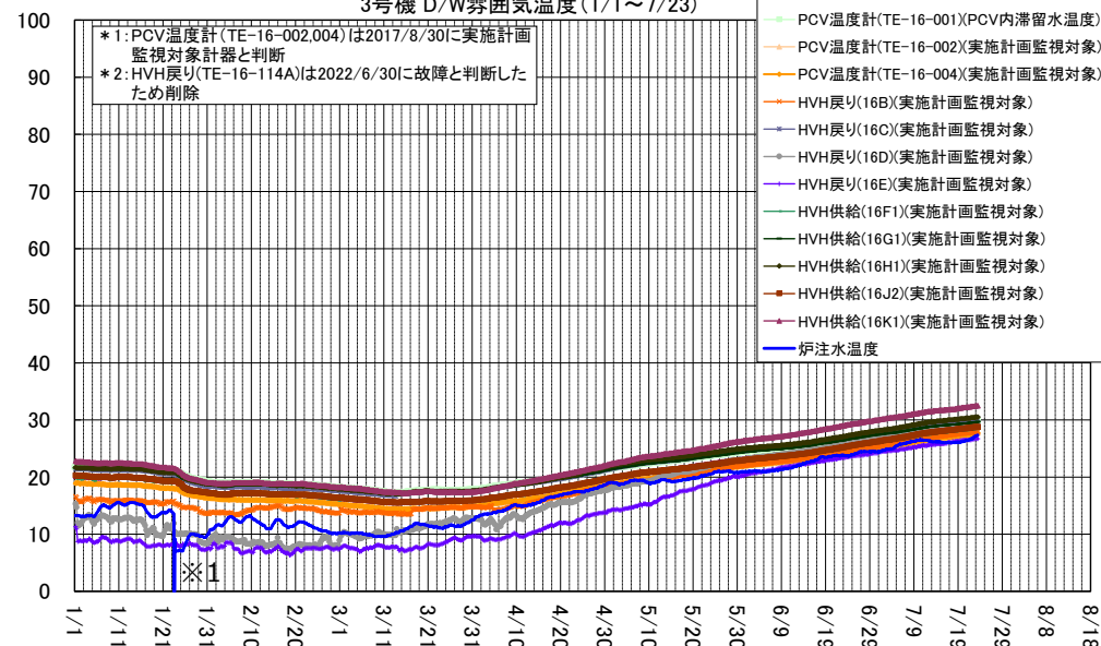
3号機 D/W雰囲気温度 (1/1~7/23)
