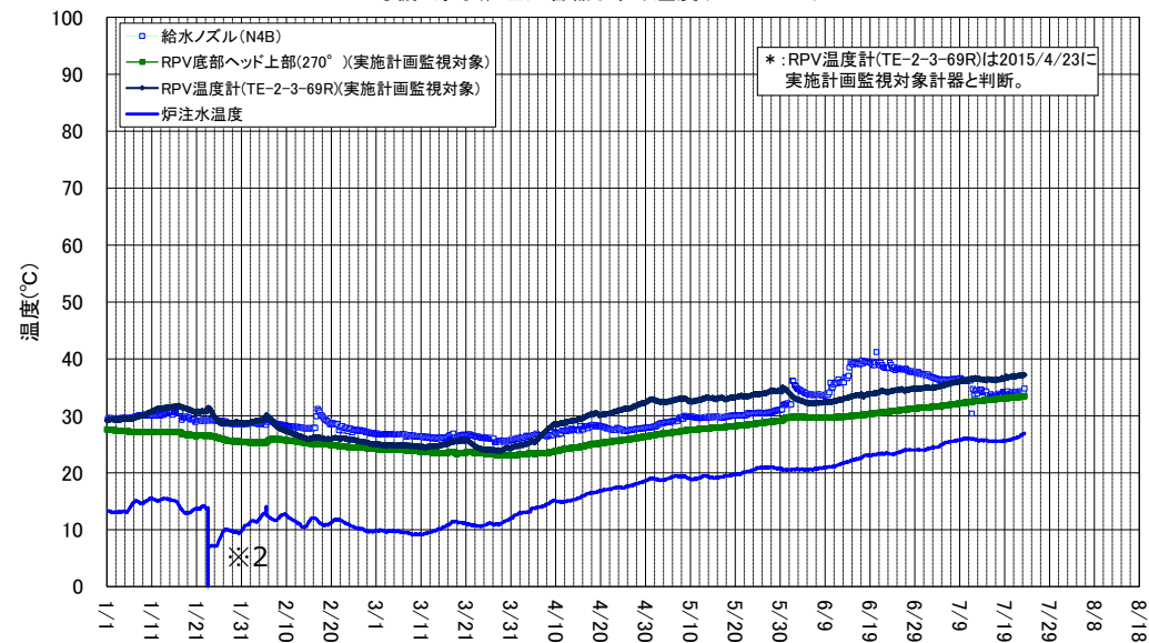
2号機 原子炉圧力容器まわり温度(1/1～7/23)
