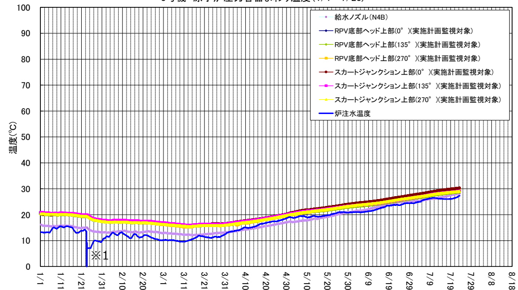
3号機 原子炉压力容器まわり温度 (1/1~7/23)
