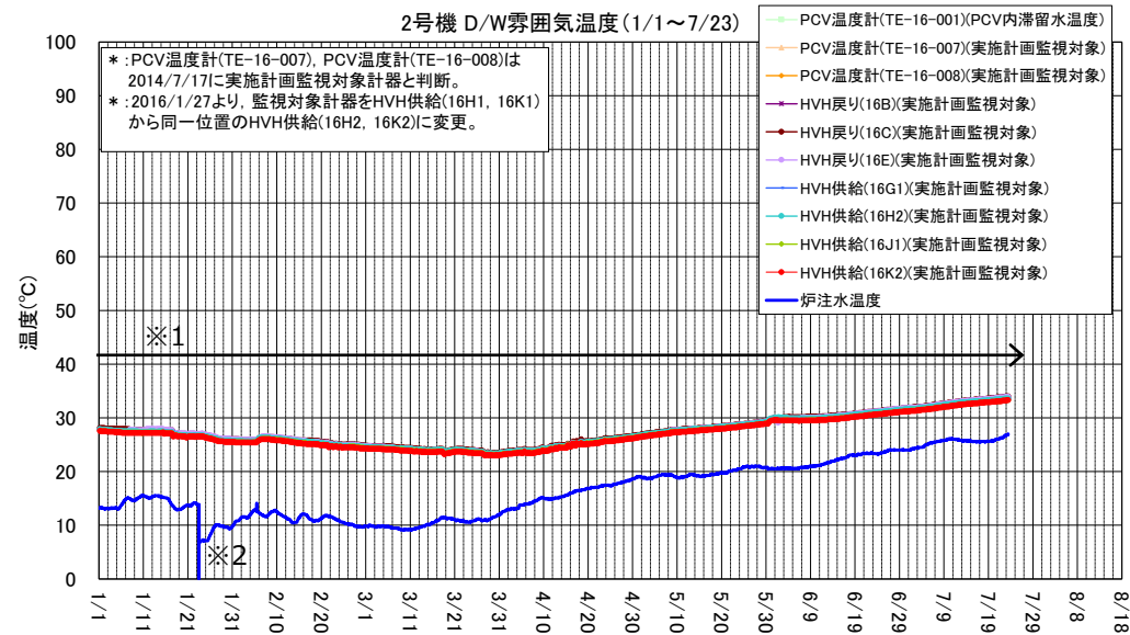
2号機 D/W雰囲気温度(1/1～7/23)
