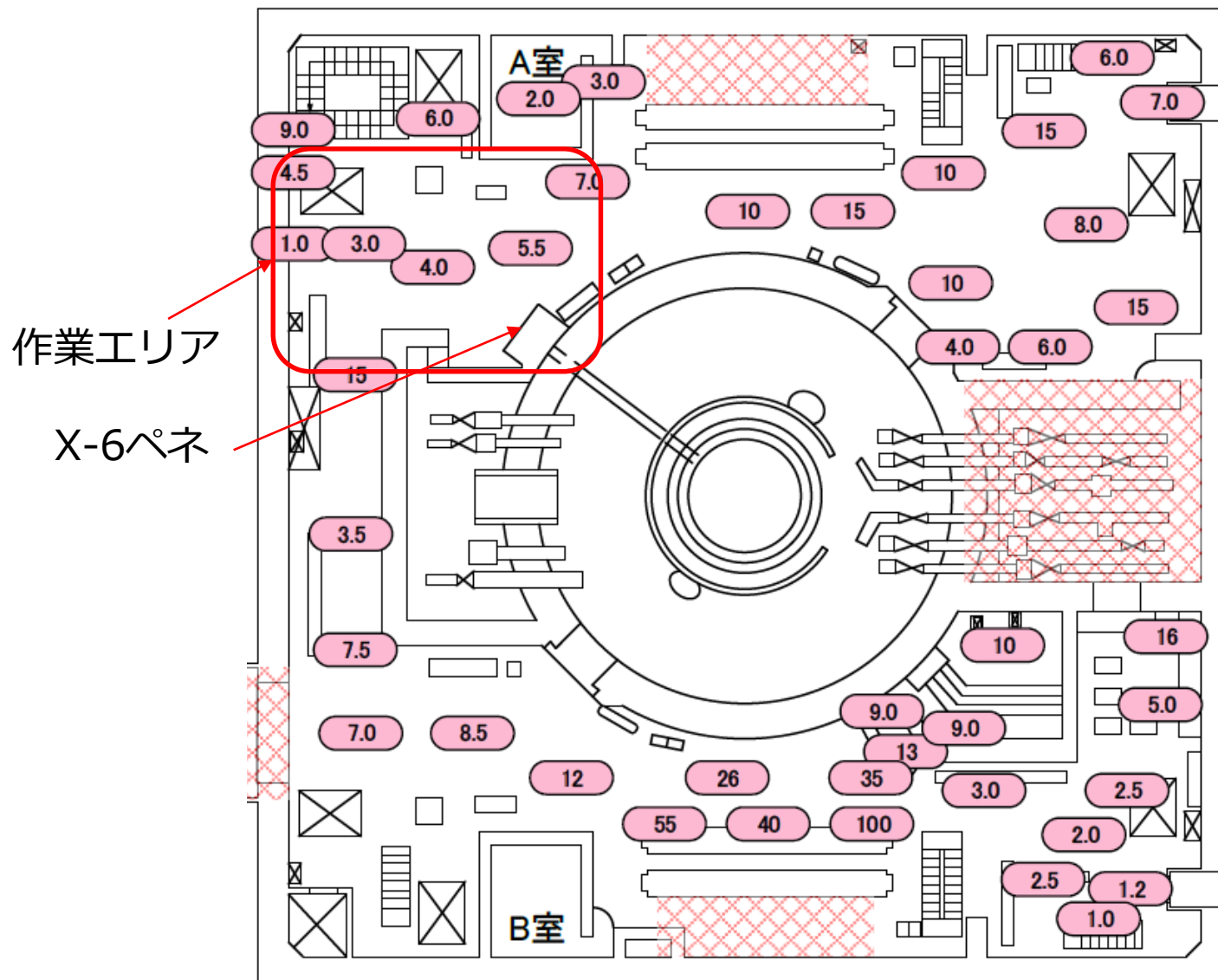
3号機R/B1階
