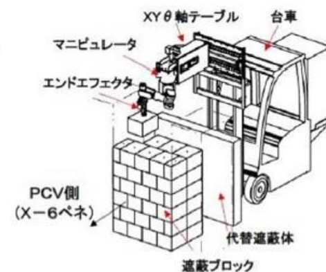
遠隔操作装置
