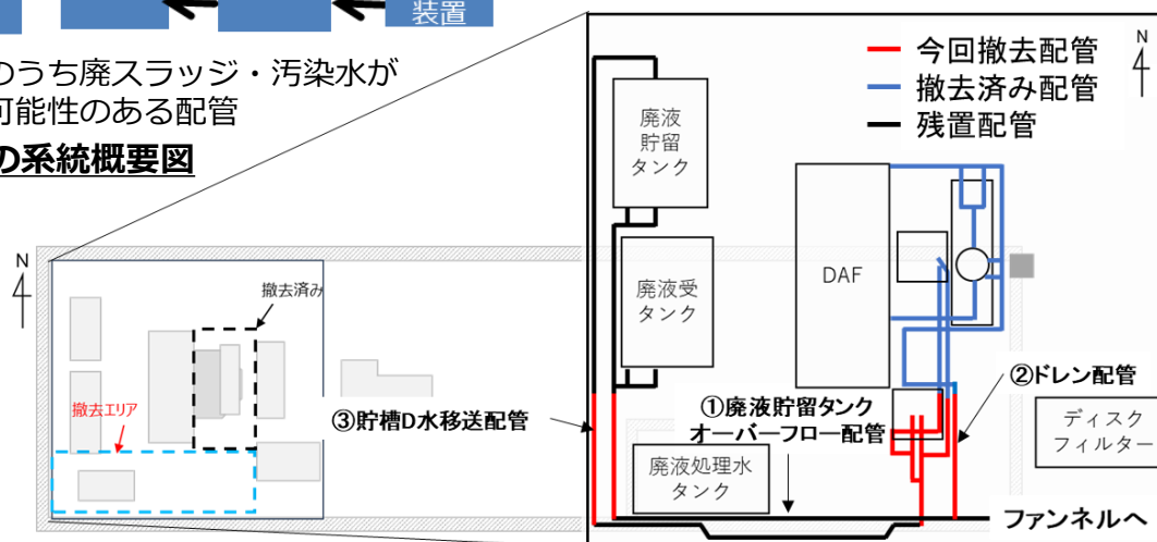
プロセス主建屋内配管撤去範囲
