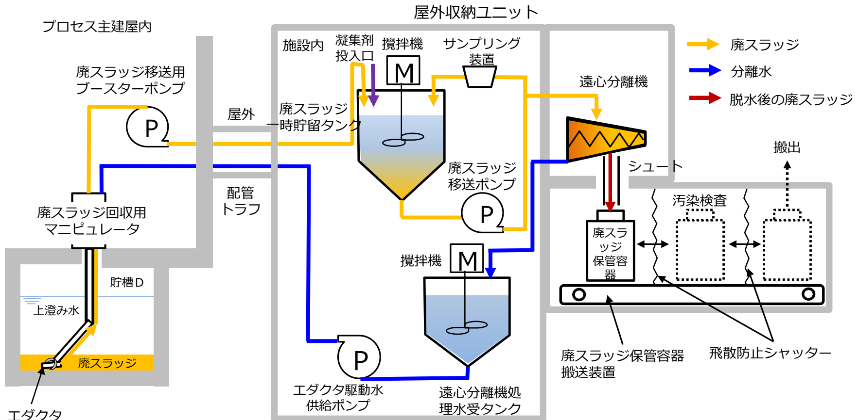
廃スラッジ回収施設系統概略図
