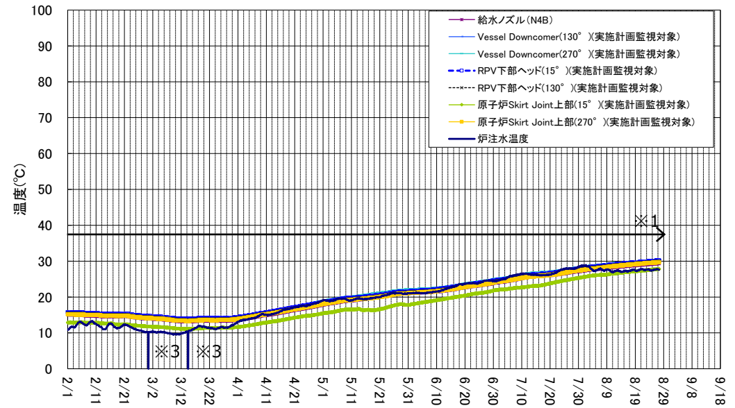
1号機 原子炉圧力容器まわり温度(2/1~8/27)
