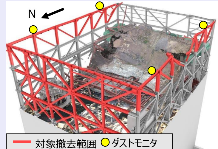
<外周鉄骨の撤去範囲>
