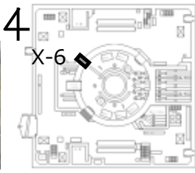
＜2号機原子炉建屋1階 ペネ配置図＞
