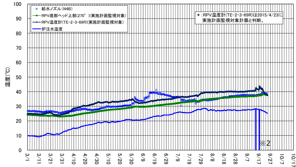
2号機 原子炉圧力容器まわり温度 (3/1～9/24)
