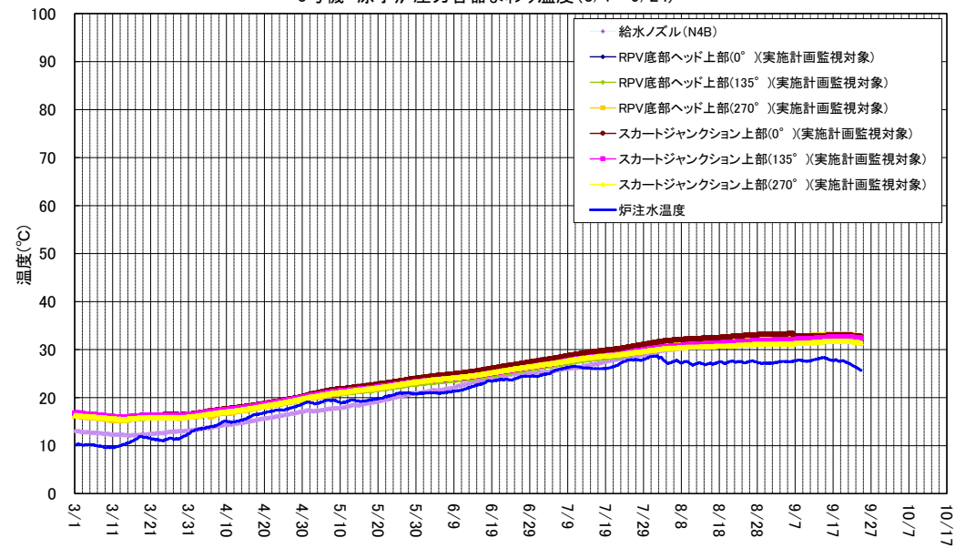
3号機 原子炉圧力容器まわり温度 (3/1~9/24)
