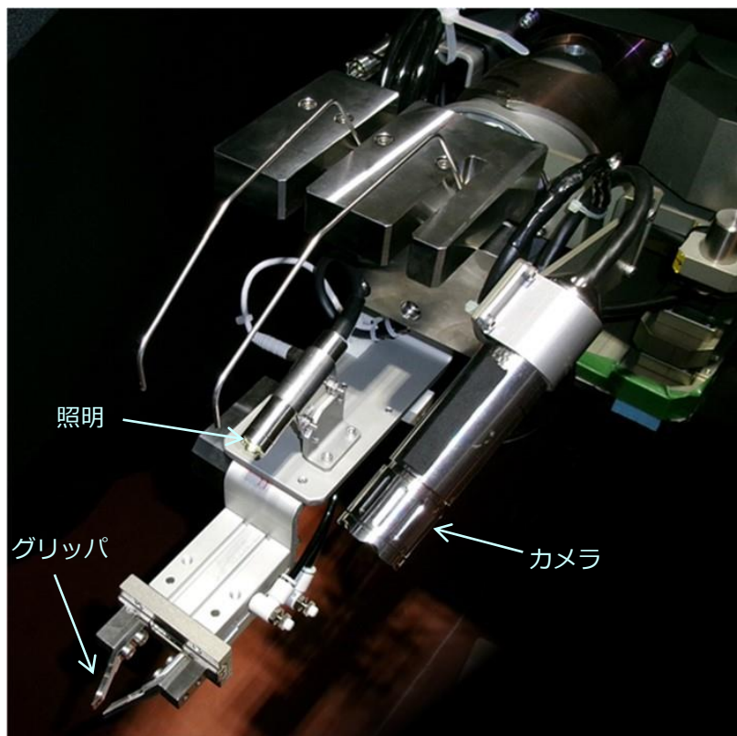
グリッパ型
