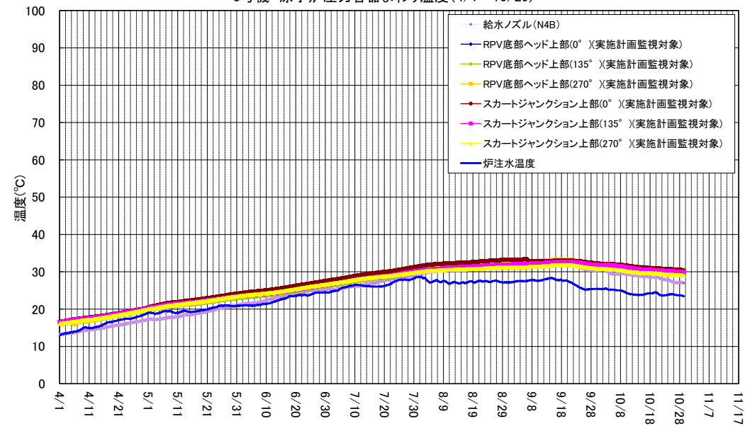
3号機 原子炉圧力容器まわり温度(4/1~10/29)
