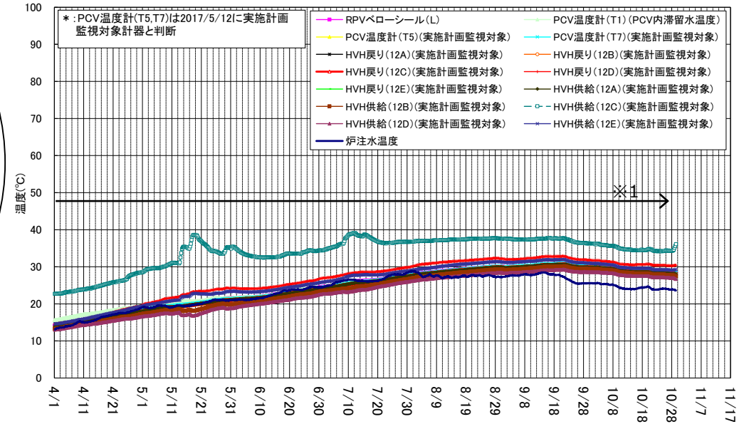
1号機 D/W雰囲気温度(4/1~10/29)
