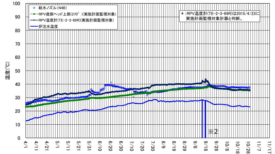
2号機 原子炉圧力容器まわり温度 (4/1～10/29)
