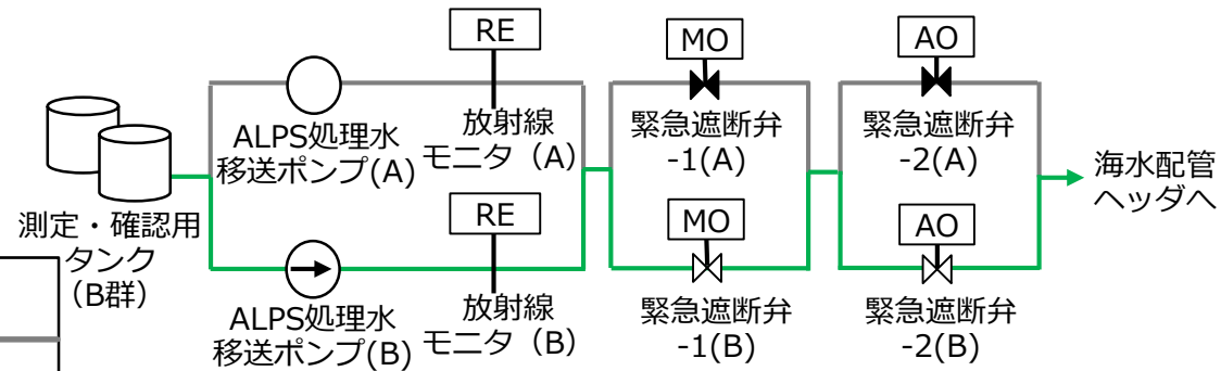
ALPS処理水移送系統図
