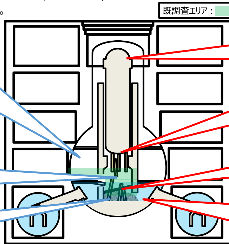
3号機原子炉建屋 縦断面概略図
