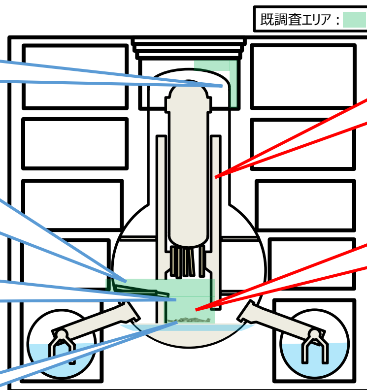
2号機原子炉建屋 縦断面概略図
