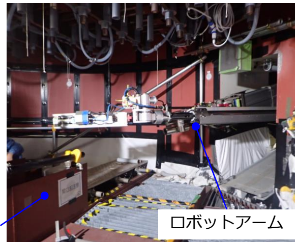
ロボットアーム櫓葉試験の状況
