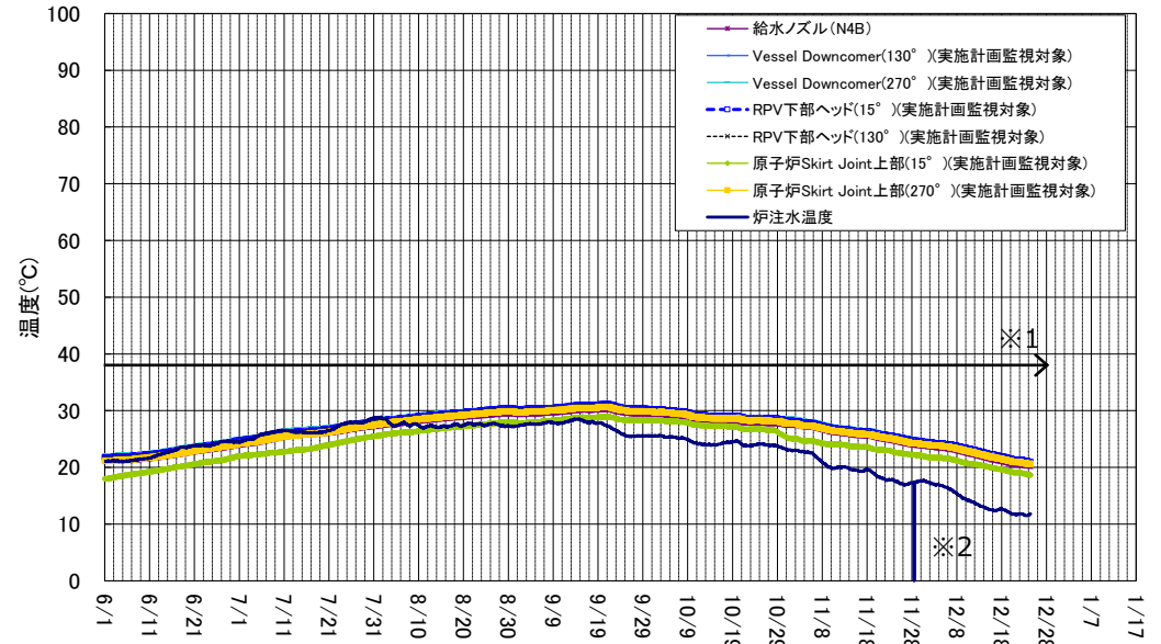
1号機 原子炉圧力容器まわり温度(6/1~12/24)
