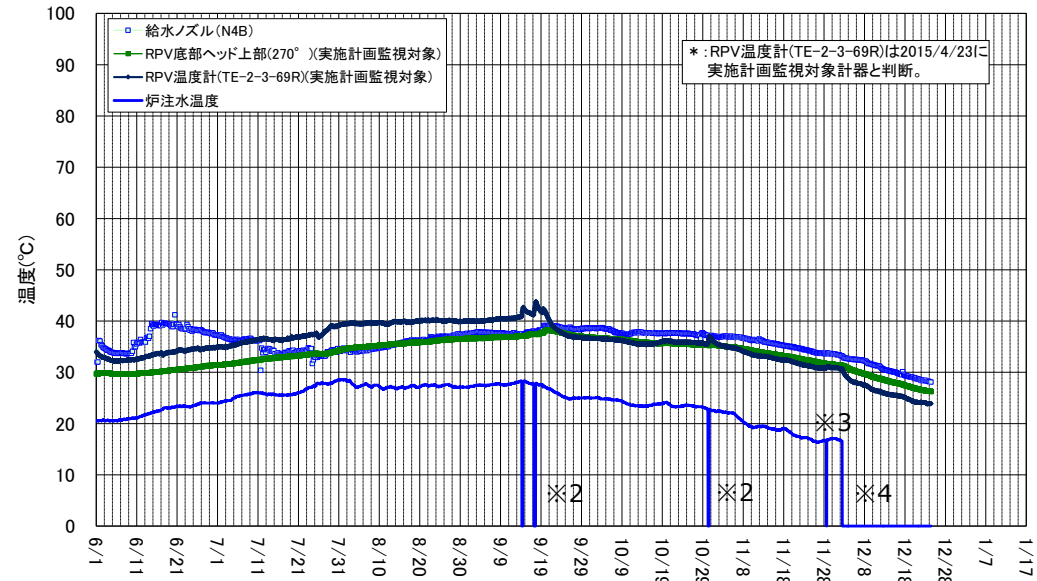
2号機 原子炉圧力容器まわり温度(6/1~12/24)
