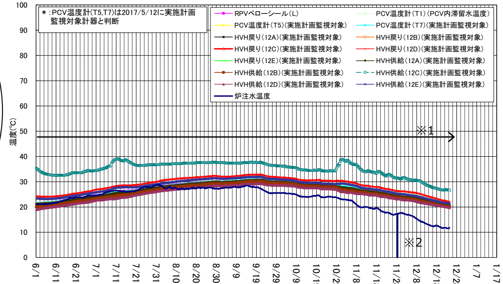
1号機 D/W雰囲気気温度(6/1~12/24)
