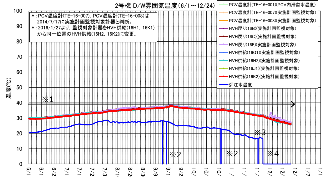
2号機 D/W雰囲気温度(6/1~12/24)
