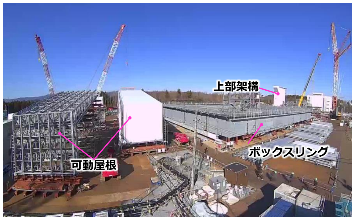
構外ヤードの状況（撮影：2月25日）
