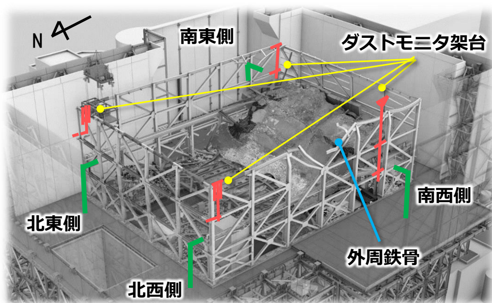
ダストモニタ架台改造の全体概要図
