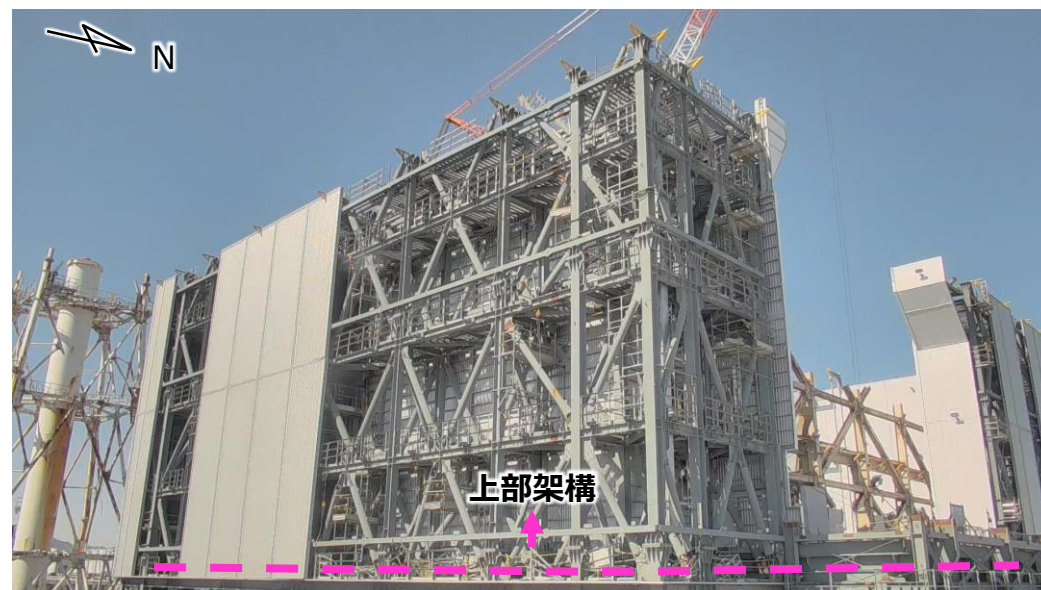
現場状況（南東面） （撮影：2月25日）
