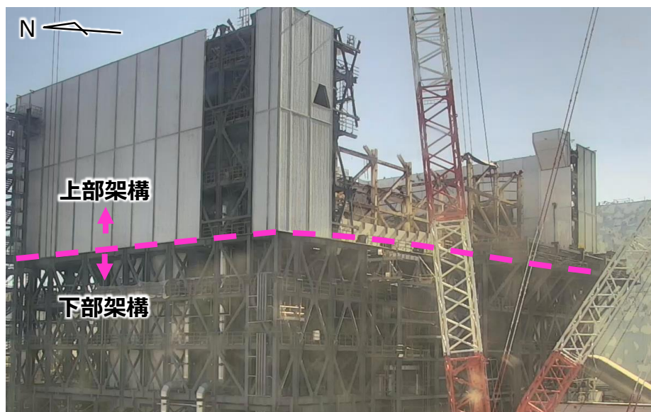
現場状況（北西面） （撮影：2月25日）
