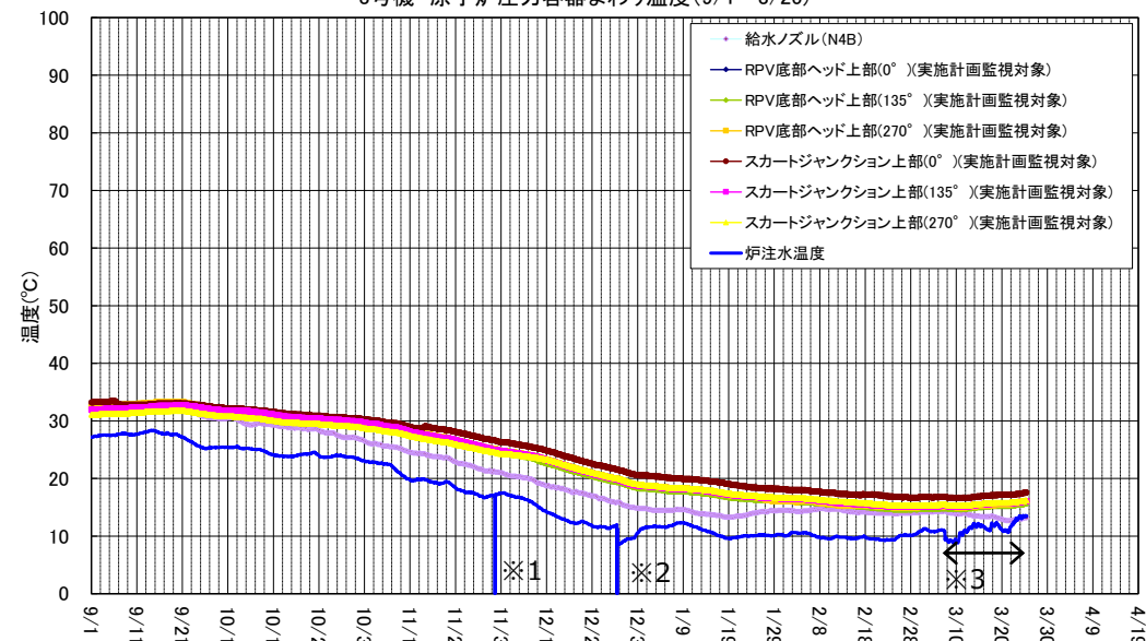
3号機 原子炉圧力容器まわり温度 (9/1~3/25)
