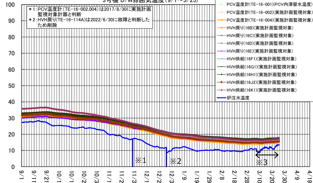
3号機 D/W雰囲気温度 (9/1~3/25)
