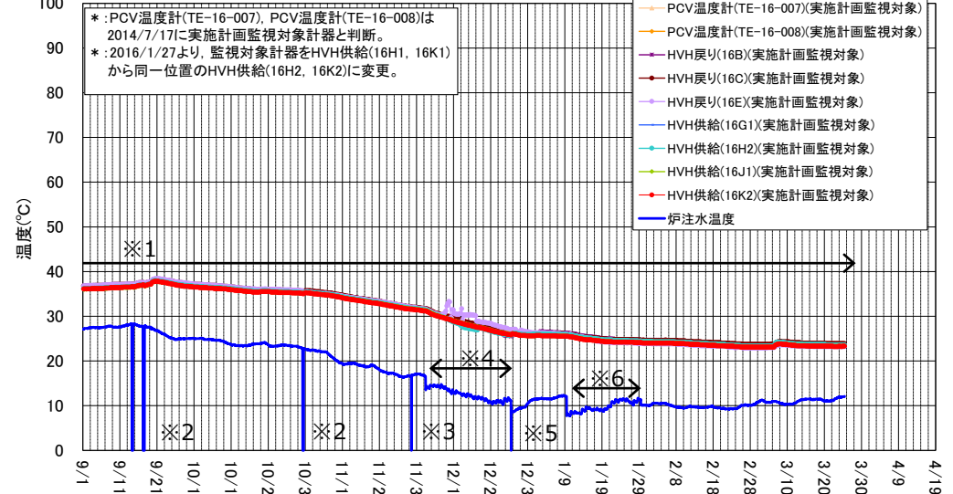
2号機 D/W雰囲気温度(9/1～3/25)
