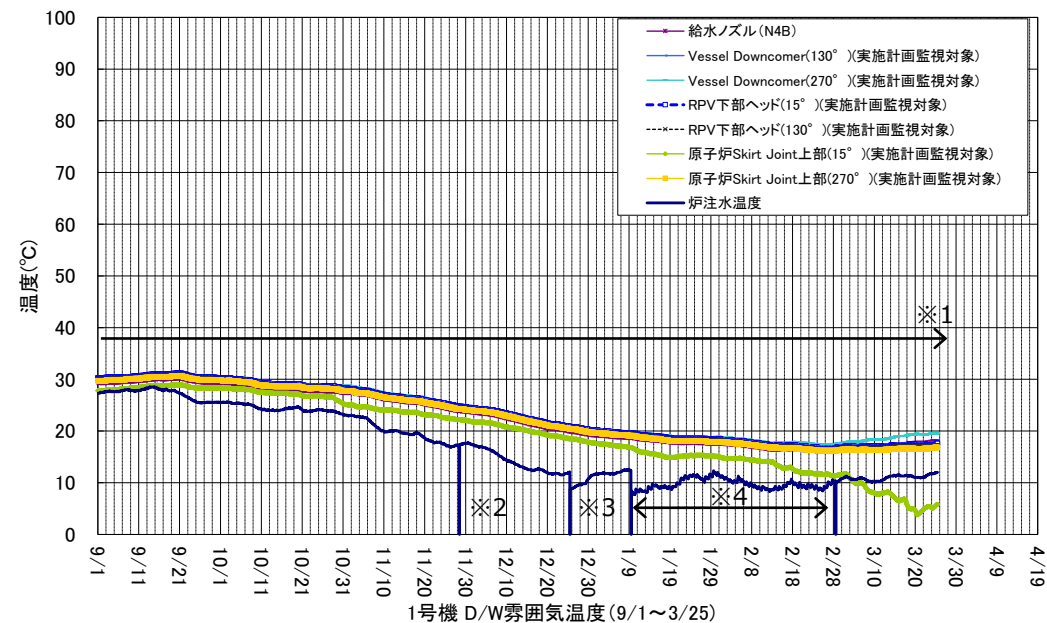
1号機 D/W雰囲気温度(9/1~3/25)
