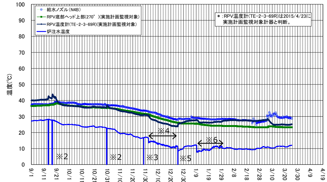
2号機 原子炉圧力容器まわり温度(9/1～3/25)
