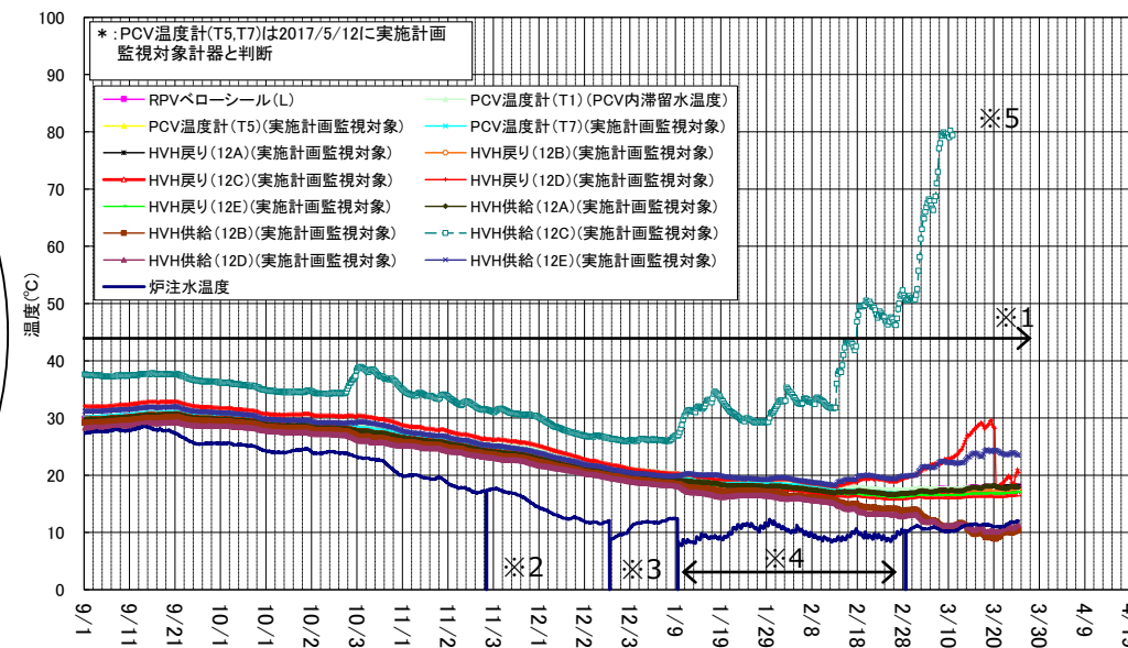
1号機 D/W雰囲気温度(9/1~3/25)
