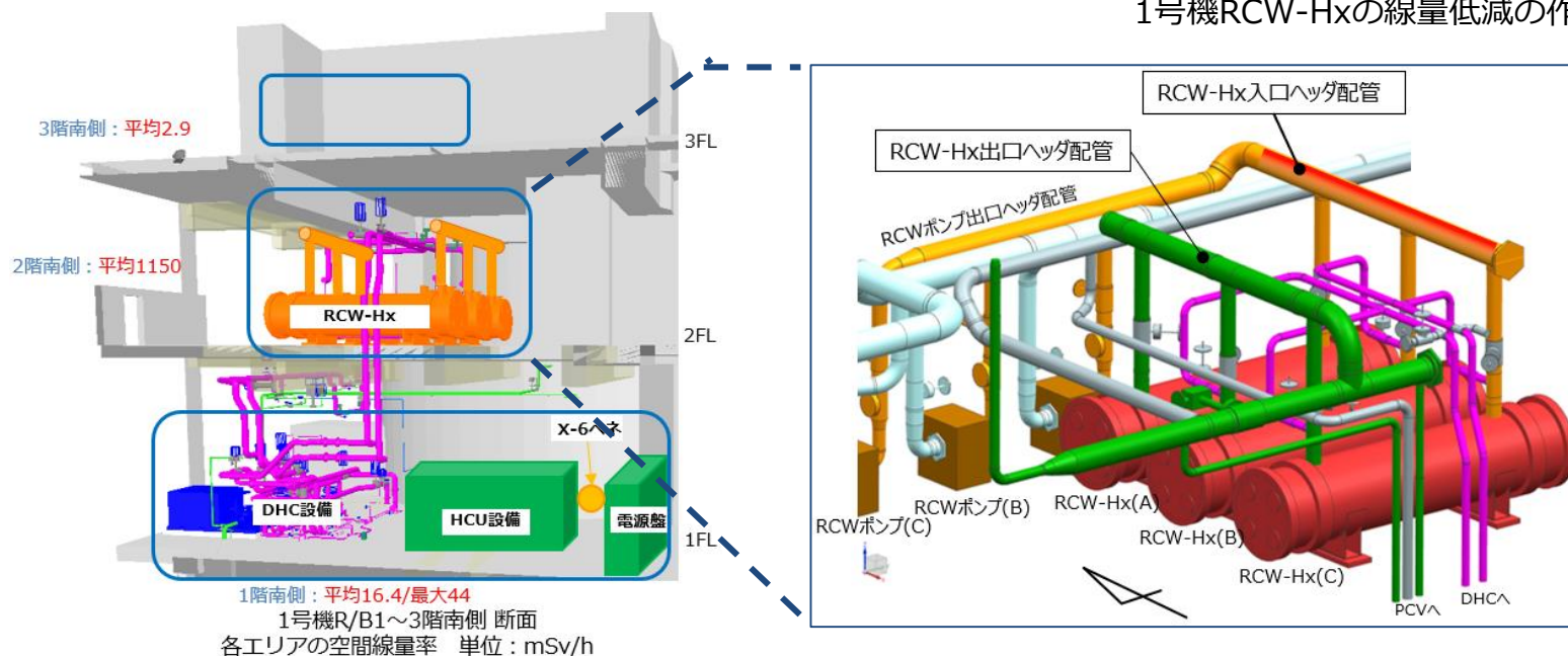
1号機RCW-Hxの配置図とR/B各階の空間線量
