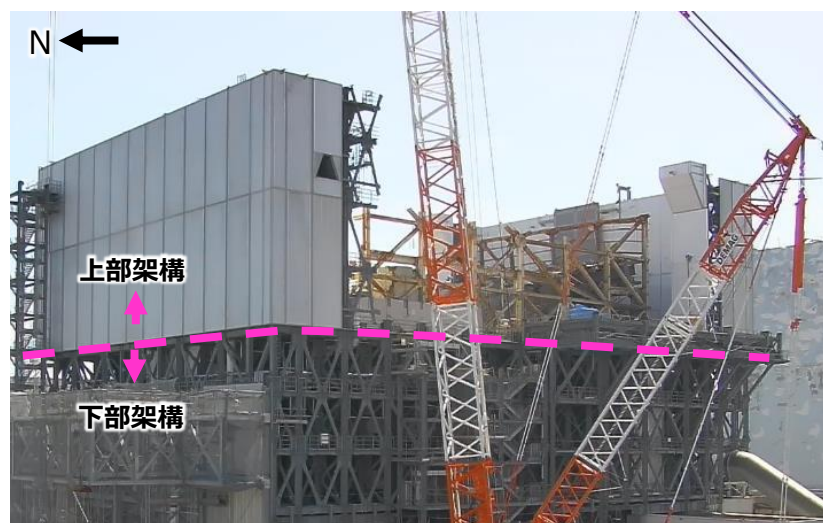
1号機大型カバー現場状況（北西側） （撮影：2025年3月18日）
