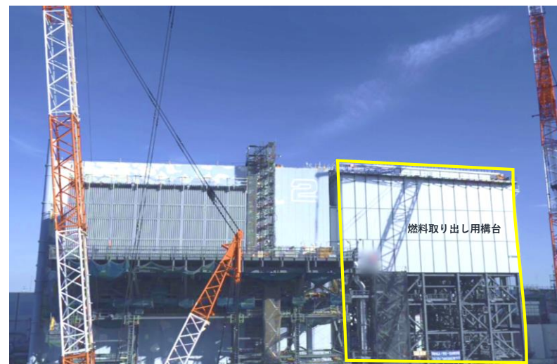
2号構台現場状況 （撮影：2024年12月3日）
