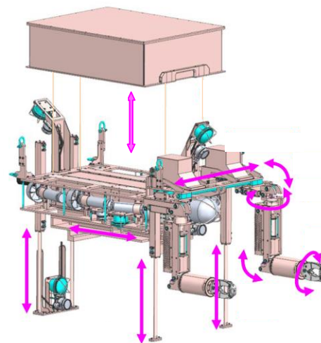
容器封入作業用ROV
