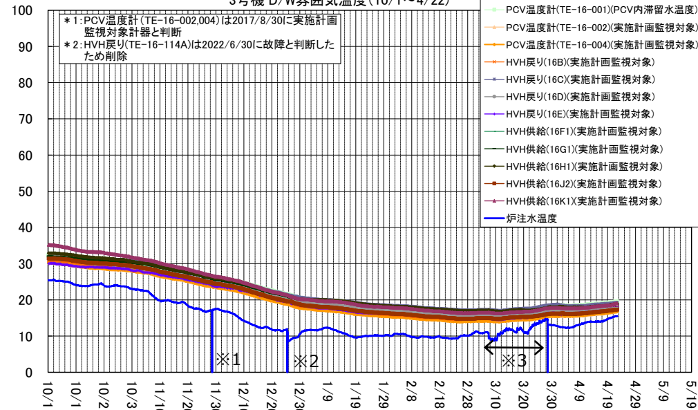
3号機 D/W雰囲気温度 (10/1~4/22)
