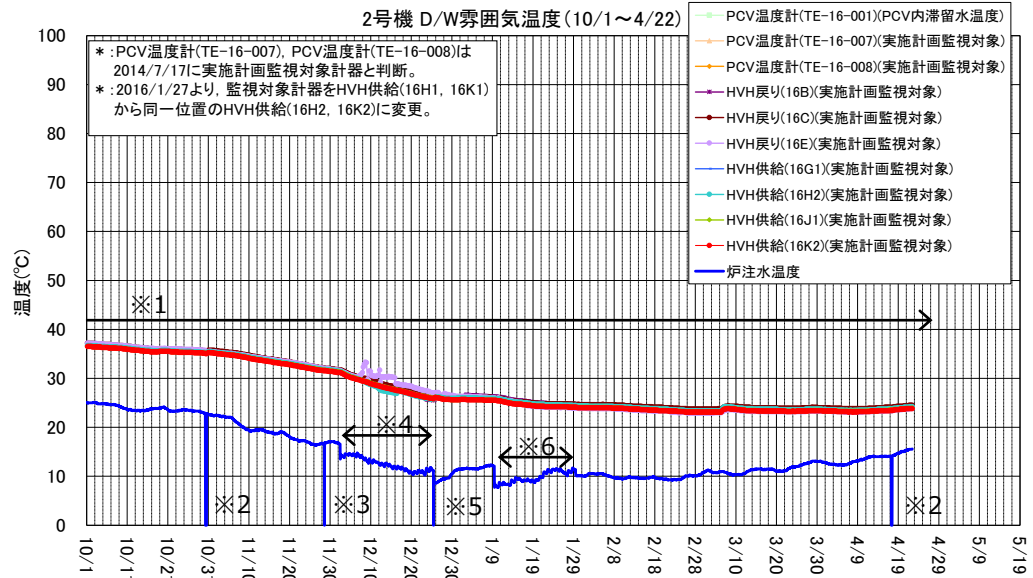
2号機 D/W雰囲気温度(10/1～4/22)
