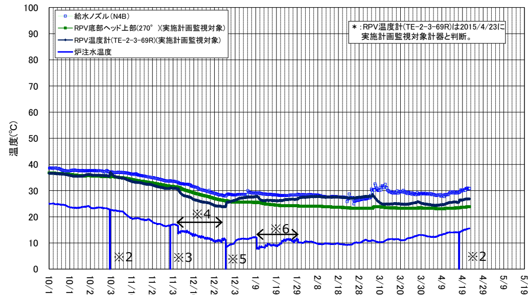
2号機 原子炉圧力容器まわり温度(10/1～4/22)
