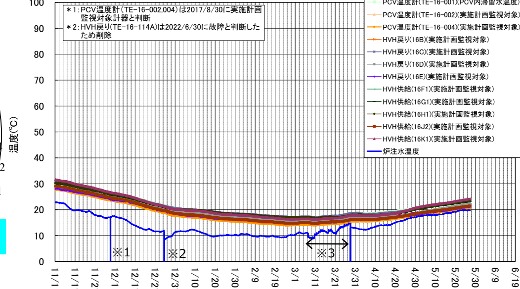
3号機 D/W雰囲気温度(11/1~5/27)
