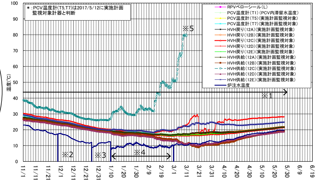
1号機 D/W雰囲気温度(11/1~5/27)
