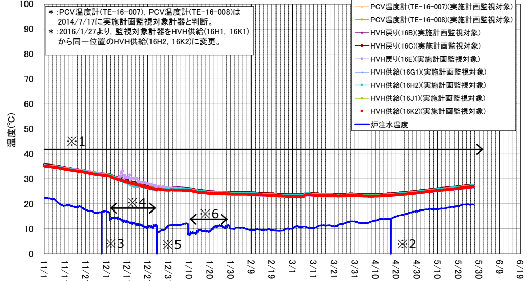
2号機 D/W雰囲気温度(11/1~5/27)
