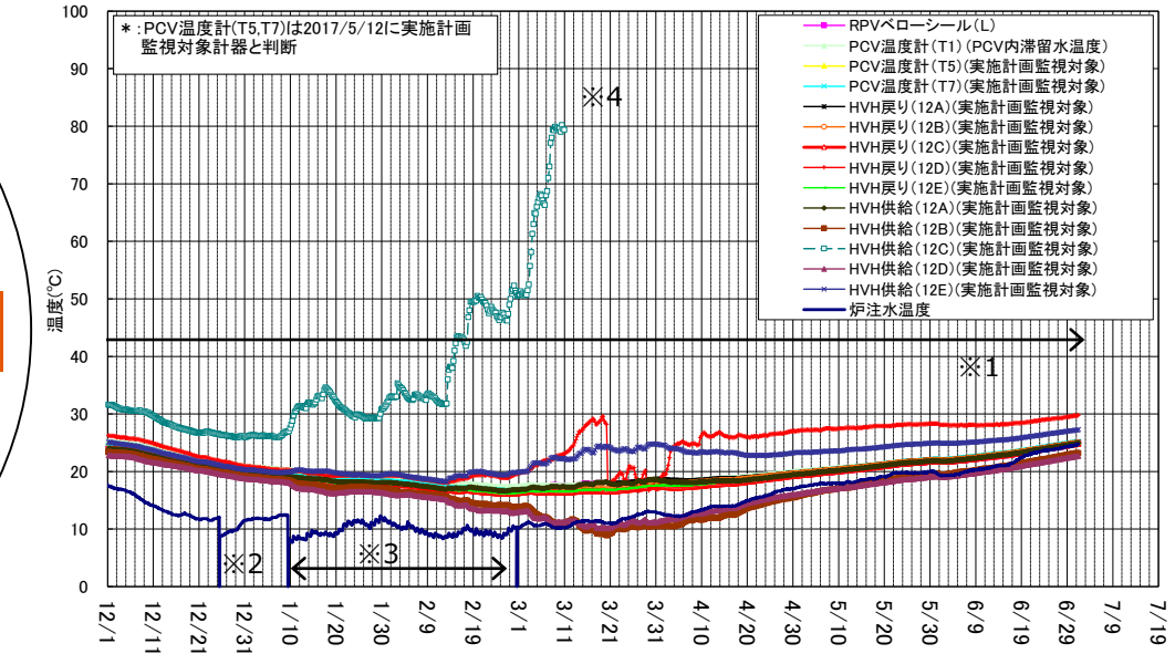
1号機 D/W雰囲気温度(12/1~7/1)
