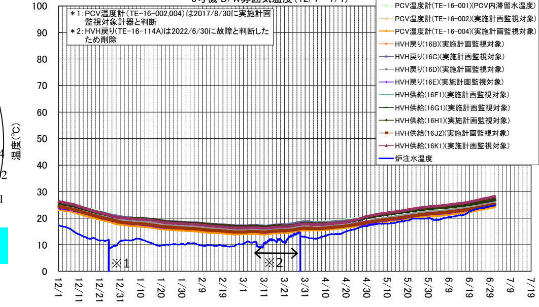
3号機 D/W雰囲気温度(12/1~7/1)
