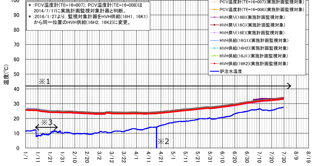
2号機 D/W雰囲気温度(1/1~7/29)
