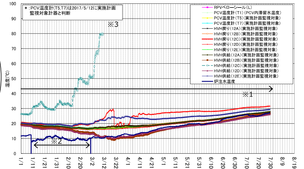
1号機 D/W雰囲気温度(1/1~7/29)
