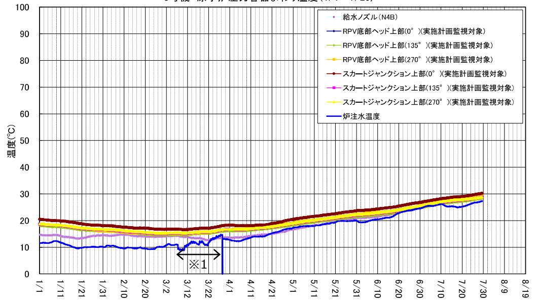
3号機 D/W雰囲気温度 (1/1~7/29)
