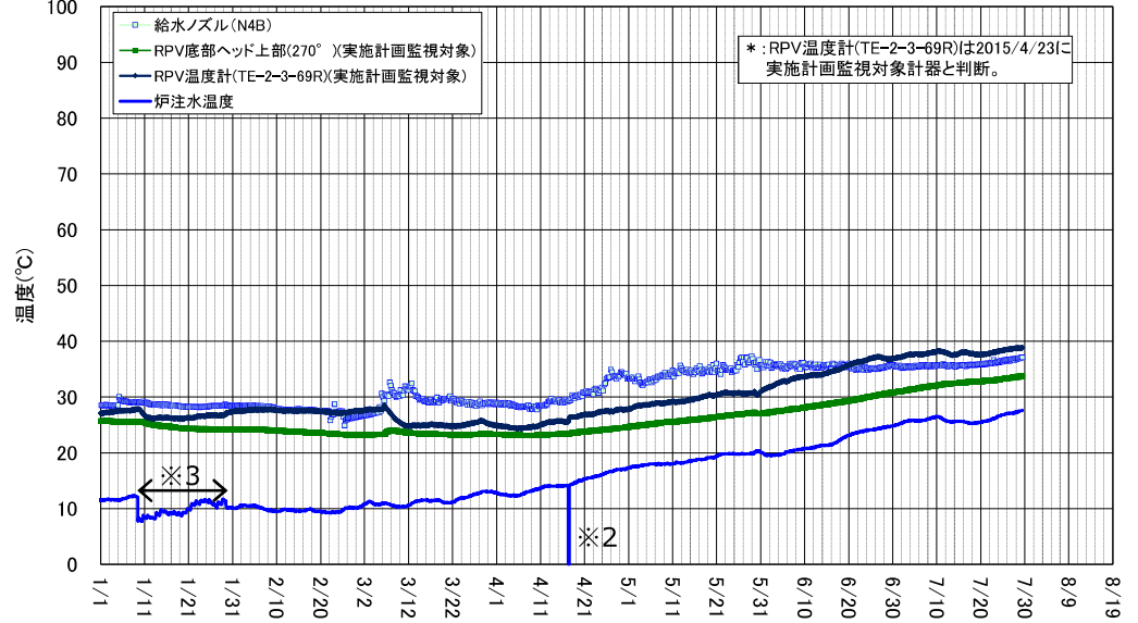
2号機 原子炉压力容器まわり温度(1/1~7/29)
