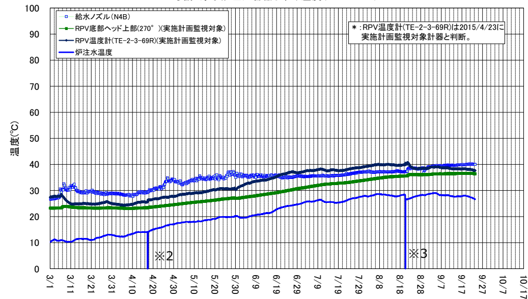
2号機 原子炉圧力容器まわり温度 (3/1～9/23)
