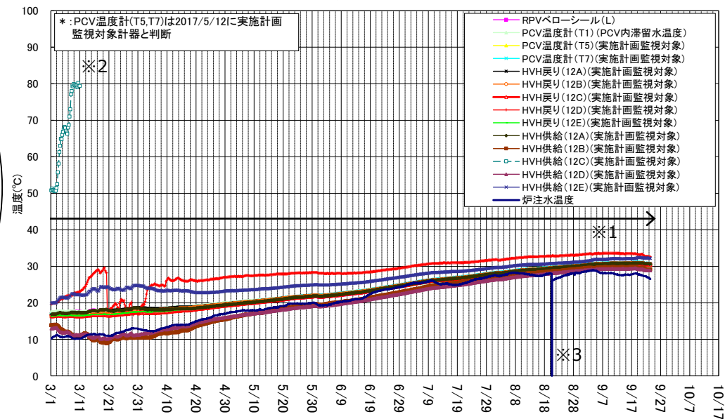
1号機 D/W雰囲気温度(3/1~9/23)
