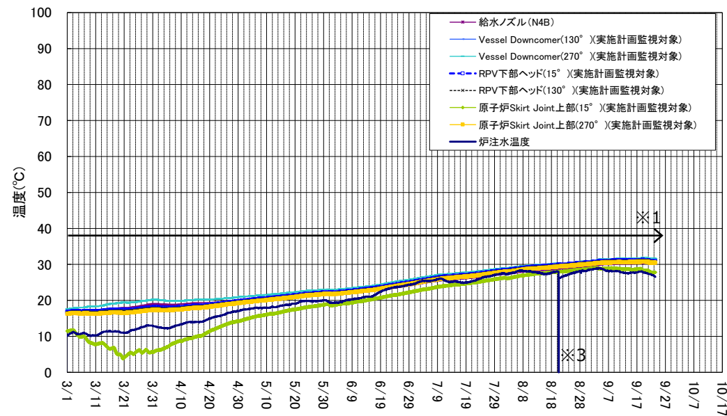
1号機 原子炉圧力容器まわり温度(3/1~9/23)
