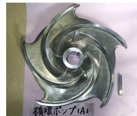
<インペラ>
