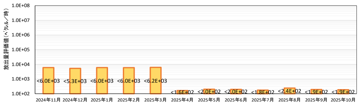
3号機 原子炉建屋、PCVガス管理システムからの放出量推移
