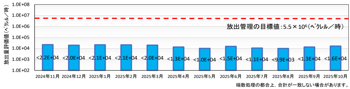
1号機 原子炉建屋、PCVガス管理システムからの放出量推移
