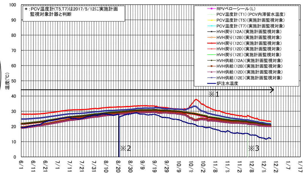
1号機 D/W雰囲気温度 (6/1~12/23)
