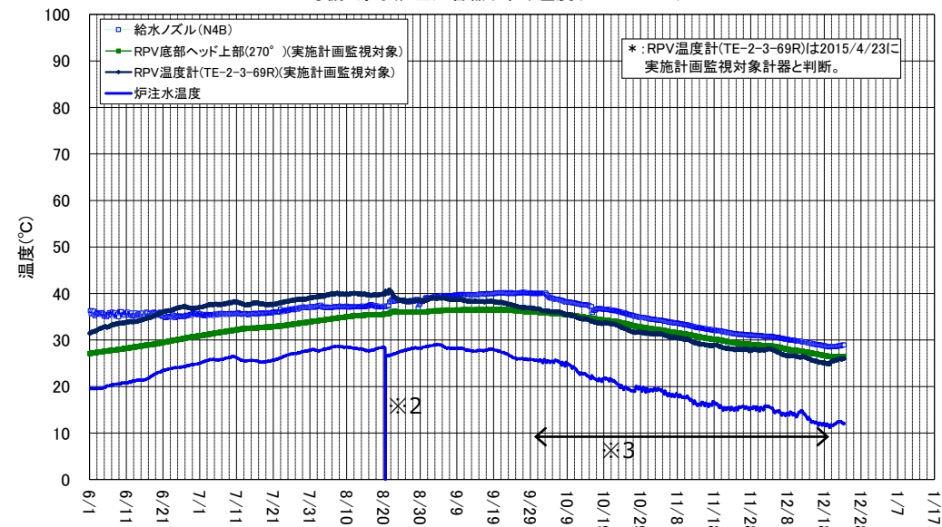
2号機 原子炉圧力容器まわり温度(6/1～12/23)
