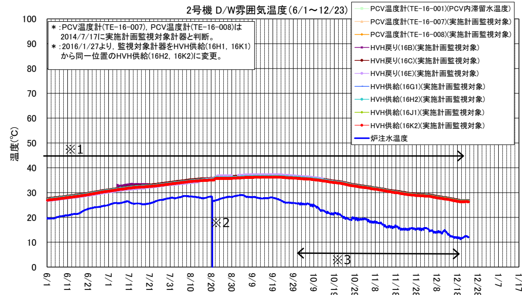
2号機 D/W雰囲気温度(6/1～12/23)
