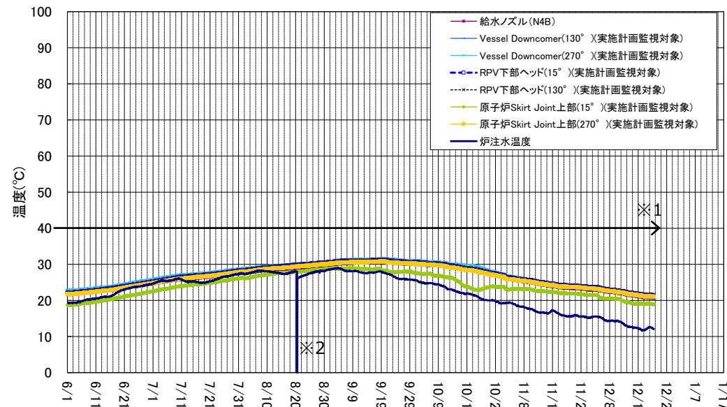
1号機 原子炉圧力容器まわり温度 (6/1~12/23)
