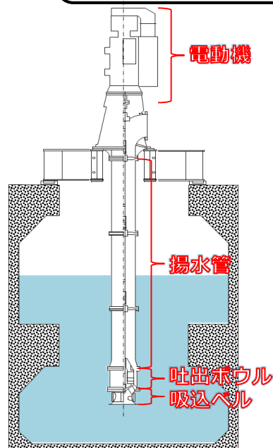
断面図
