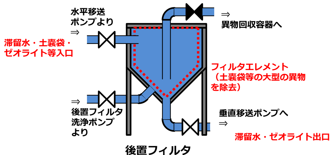
異物回収フィルタ（後置フィルタ）
