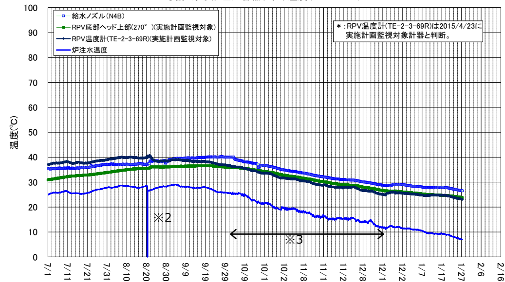
2号機 原子炉圧力容器まわり温度(7/1～1/27)
