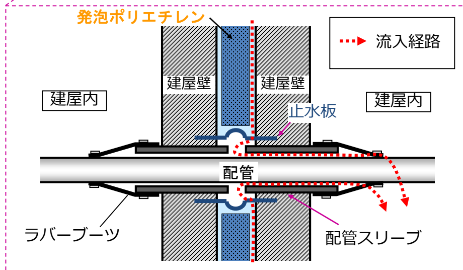
建屋間断面図
