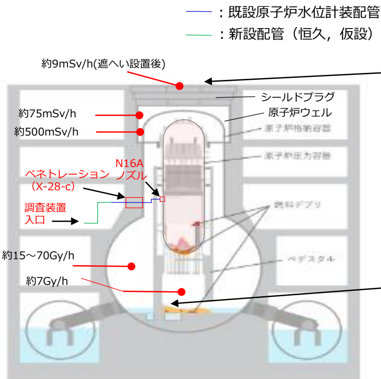
2号機原子炉建屋の状況 (RPV内は未確認)
