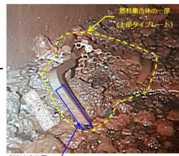
RPV外で確認された燃料集合体の一部 (上部タイプレート)
