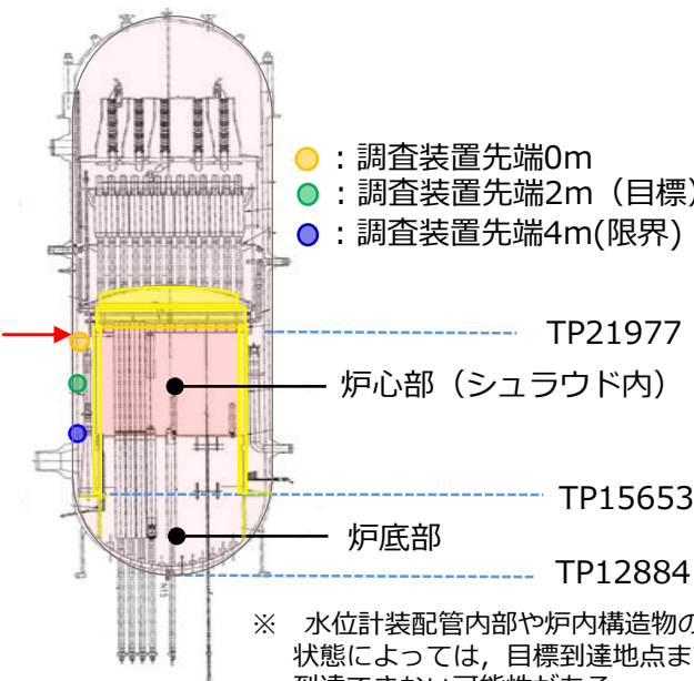
炉内構造物と調査範囲
