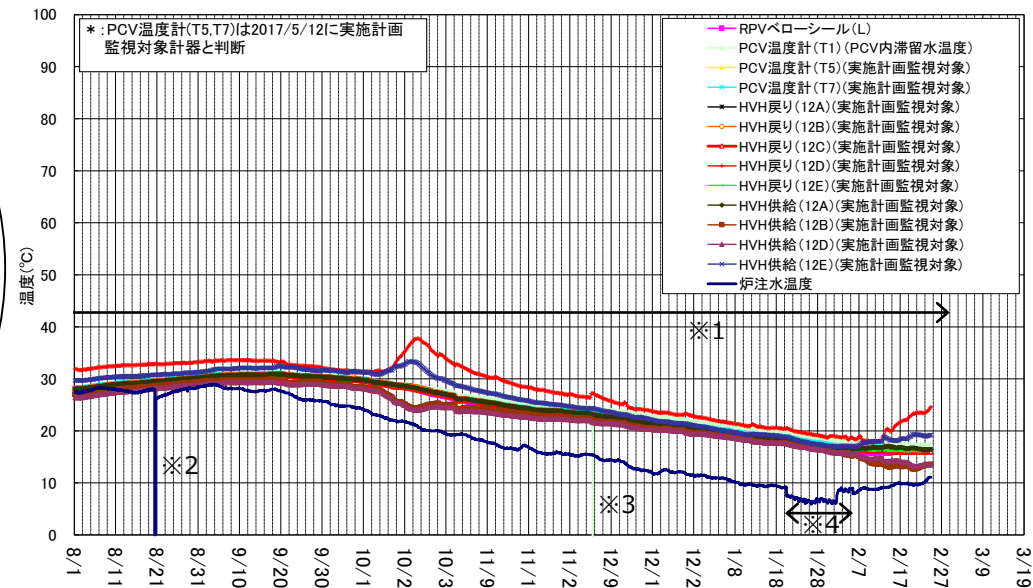
1号機 D/W雰囲気温度 (8/1～2/24)
