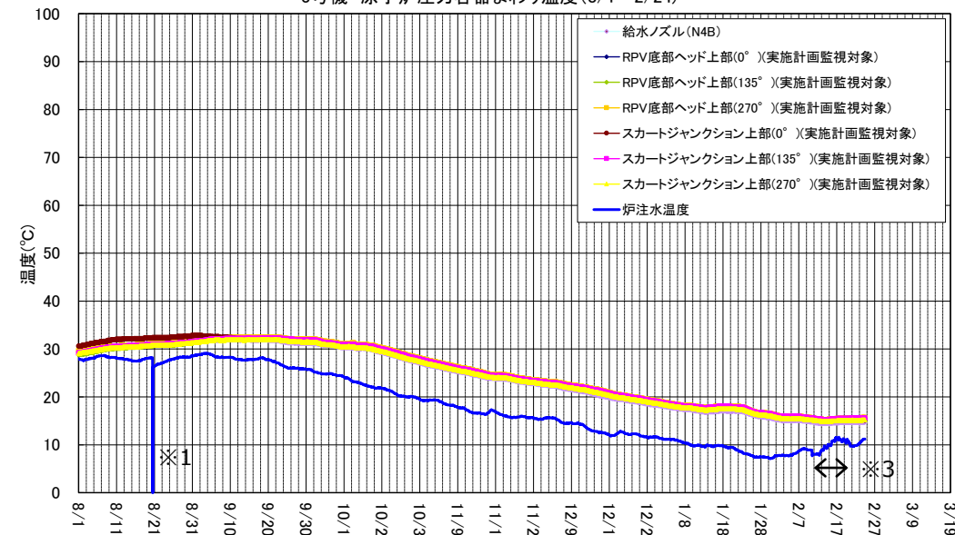
3号機 原子炉圧力容器まわり温度 (8/1~2/24)
