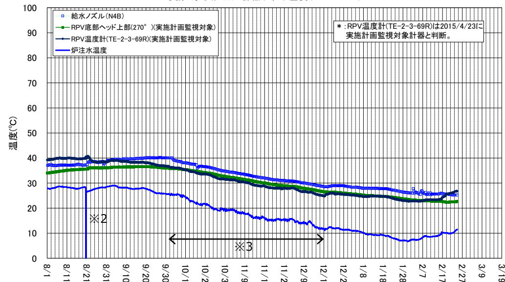
2号機 原子炉圧力容器まわり温度(8/1～2/24)
