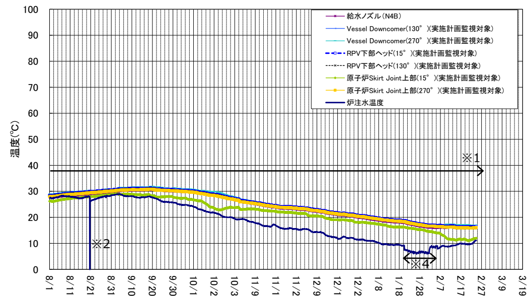
1号機 原子炉圧力容器まわり温度 (8/1～2/24)
