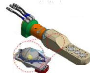
ガンマ線量
