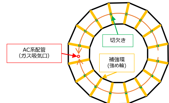
3号機S/C平面図 (補強環配置イメージ)
