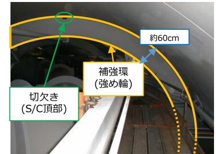
3号機S/C補強環（震災前のS/C内部）
