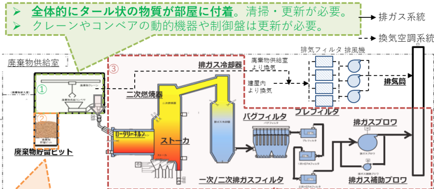
増設雑固体廃棄物焼却設備の概要
