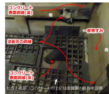
貯留ピットの状況（チップ・水回収後）
